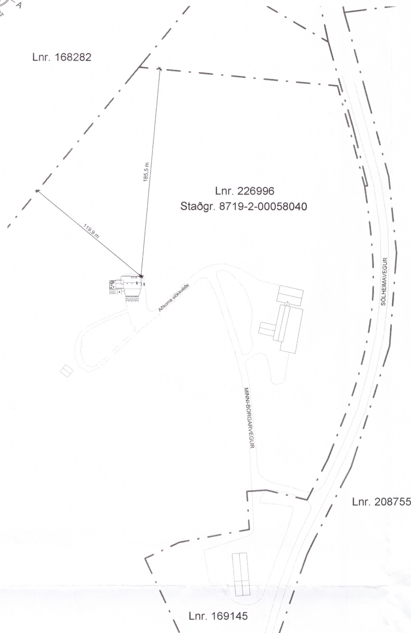
Afstöðumynd 1 : 2000
