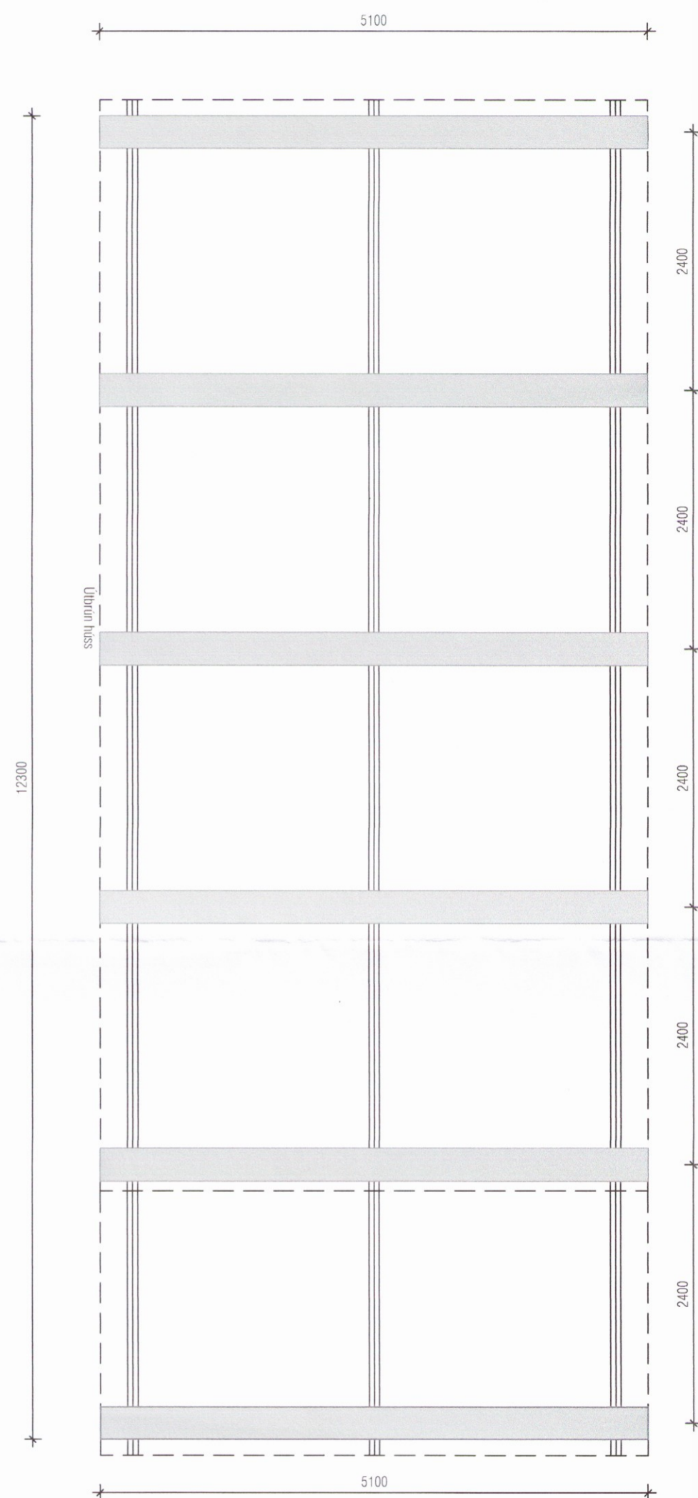
UNDIRSTÖÐUR - GRUNNMYND 1:50
