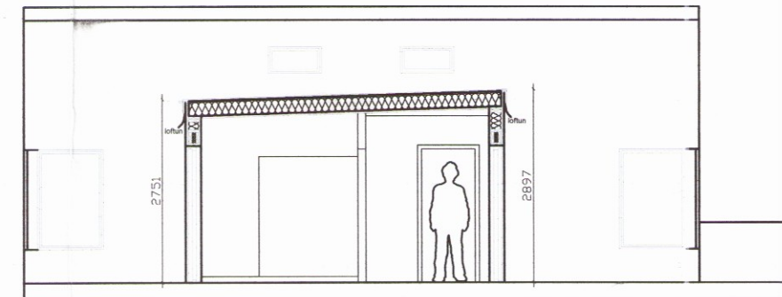
Snið B-B
