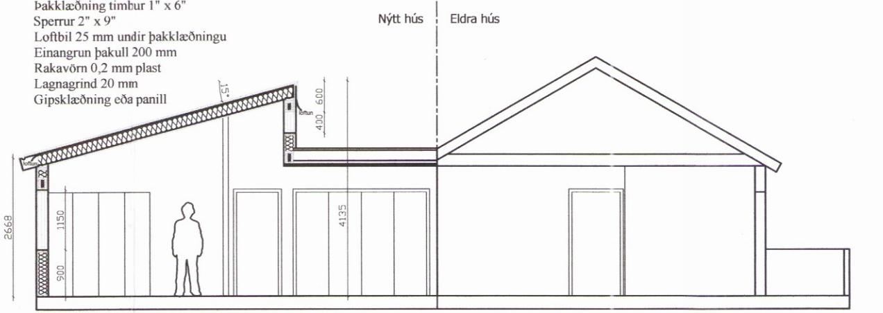
Snið A-A
