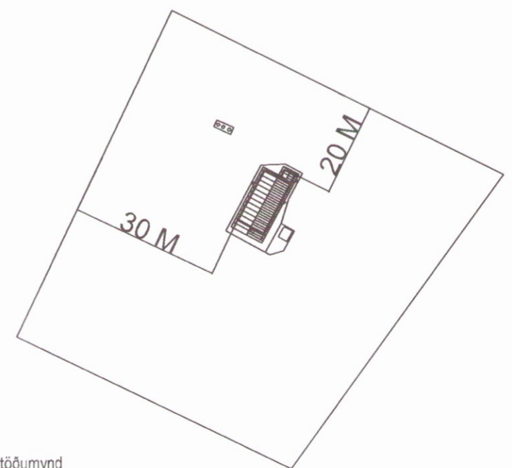
Afstöðumynd 1:1000
