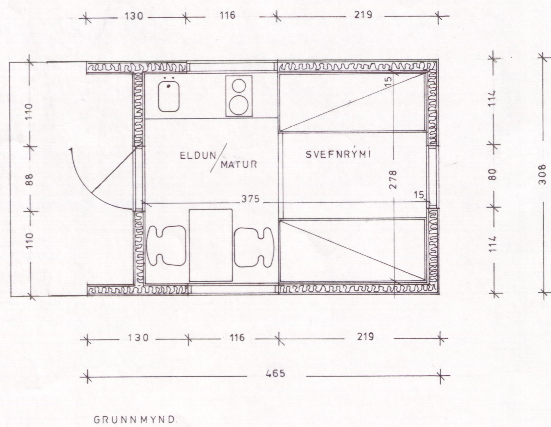
GRUNNMYND
