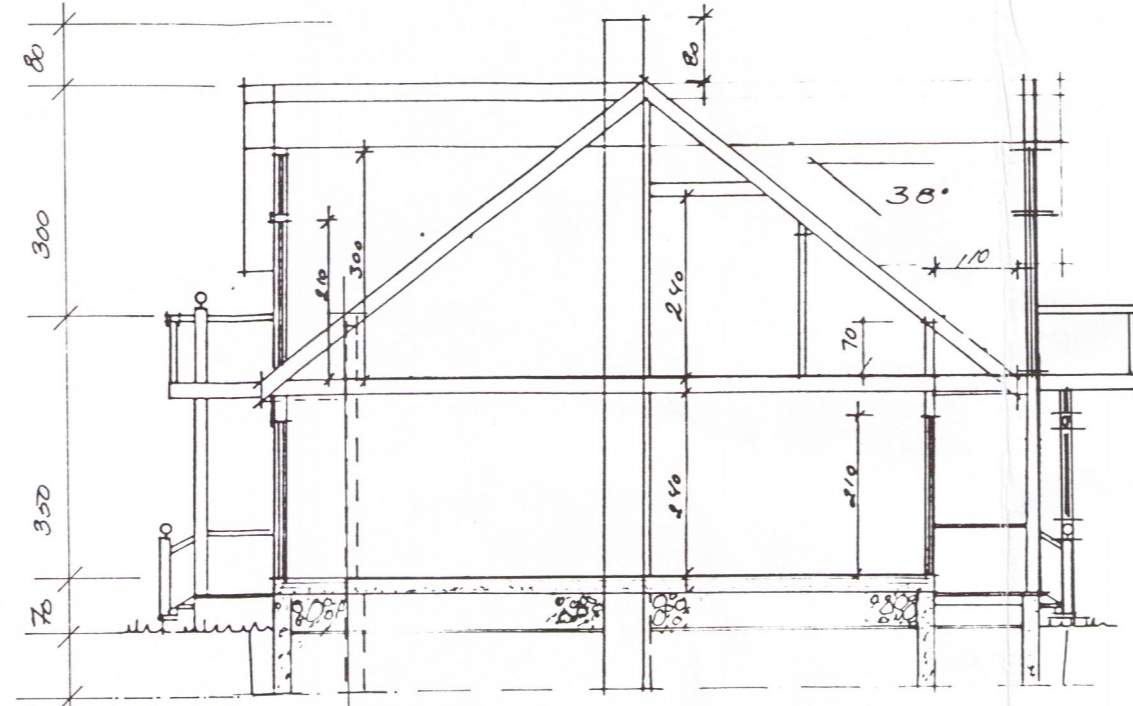
SNEIDING A-A
