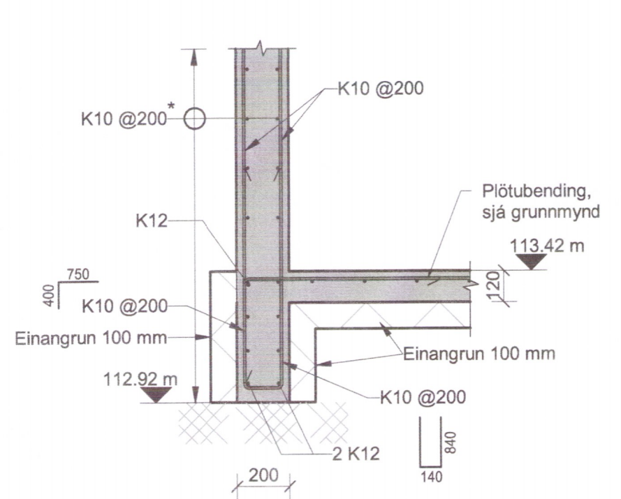
AA Snið AA 01_1_21_01 1 : 20
