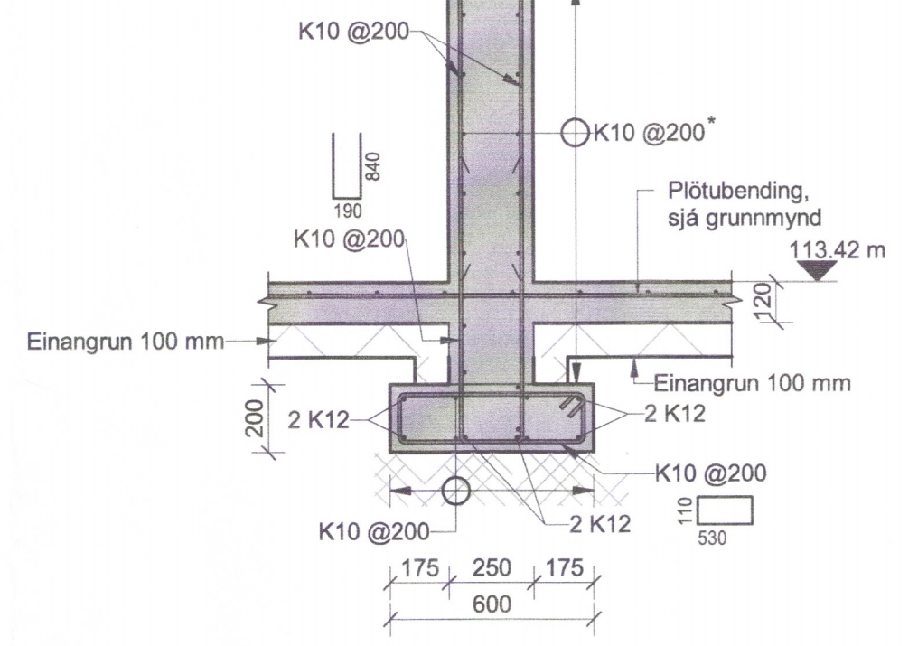
AD Snið AD 01_1_21_01 1 : 20
