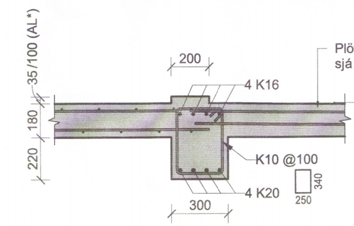
AL Snið AL 01_1_21_01 1 : 20 Snið AL* er sambærilegt nema steypur kantur er 100 mm upp úr
