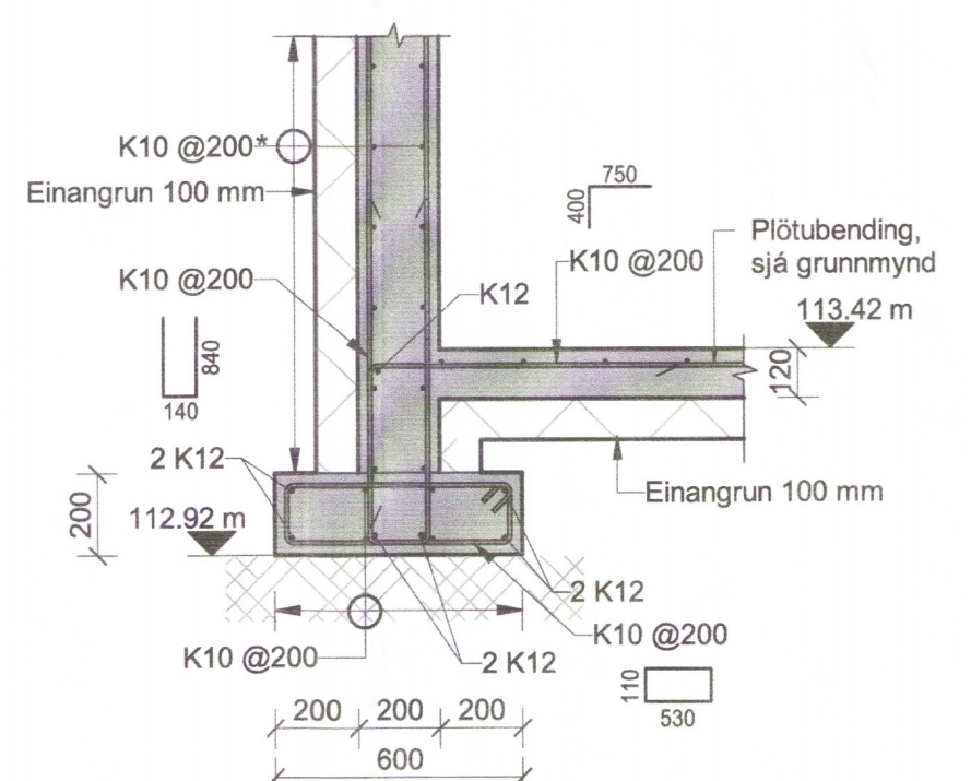
AB Snið AB 01_1_21_01 1 : 20
