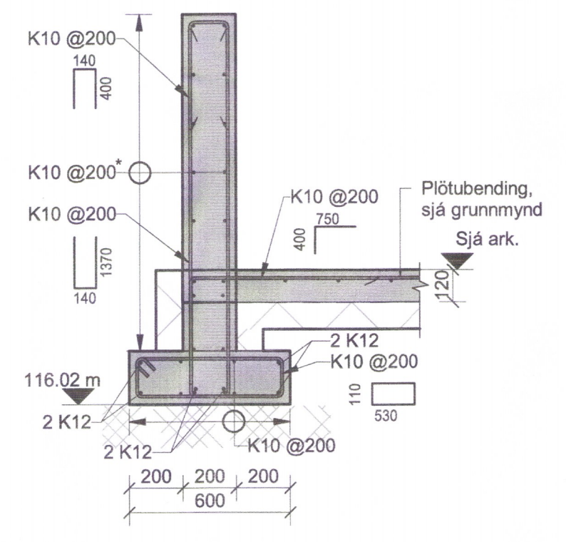
AQ Snið AQ 01_1_21_01 1 : 20
