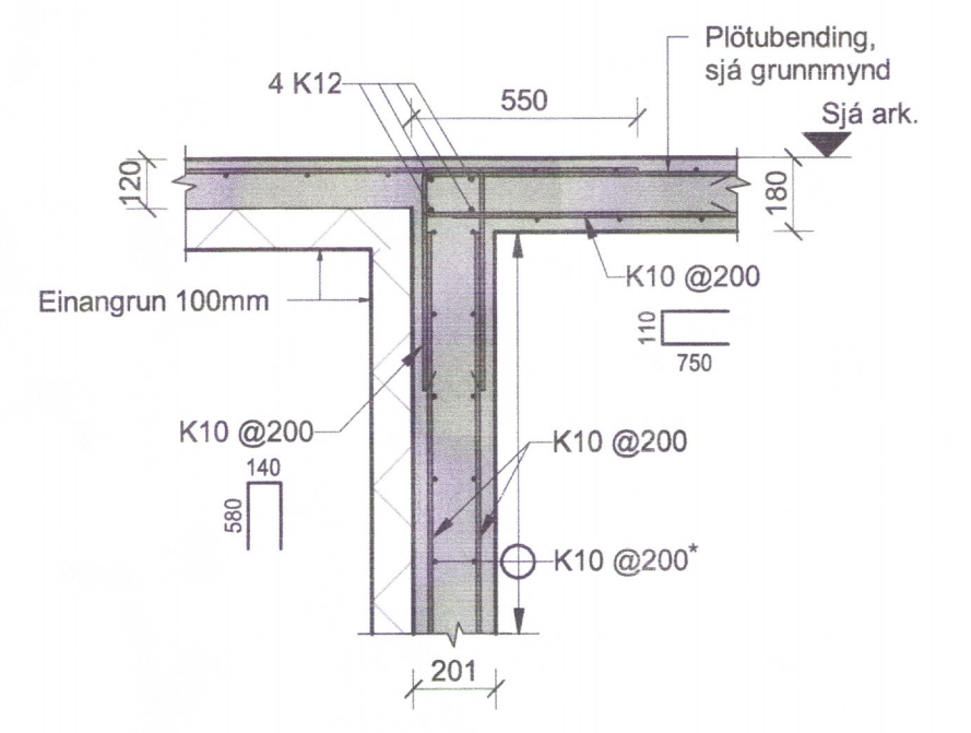
AJ Snið AJ 00_1_21_01 1 : 20
