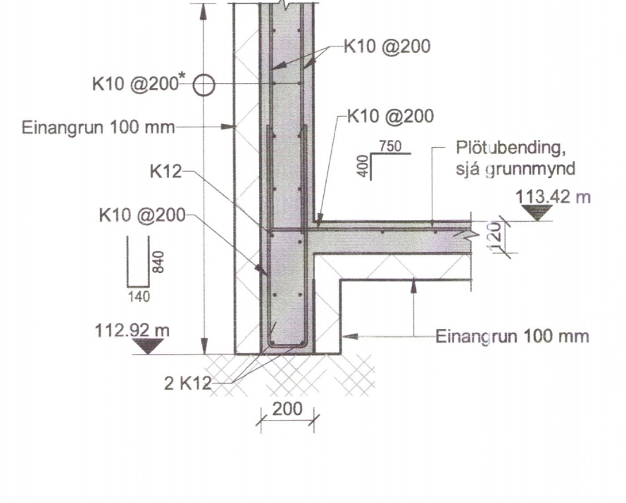
AC Snið AC 01_1_21_01 1 : 20
