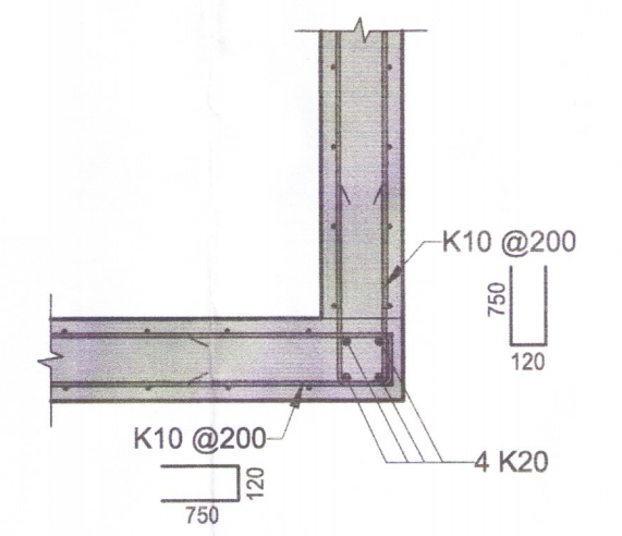
BC Deili BC 00_1_21_01 1 : 20
