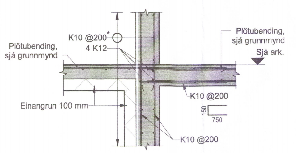
AP Snið AP 01_1_21_01 1 : 20
