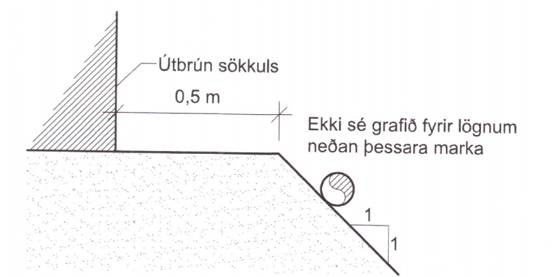
Legu lagna við hús 1:20
