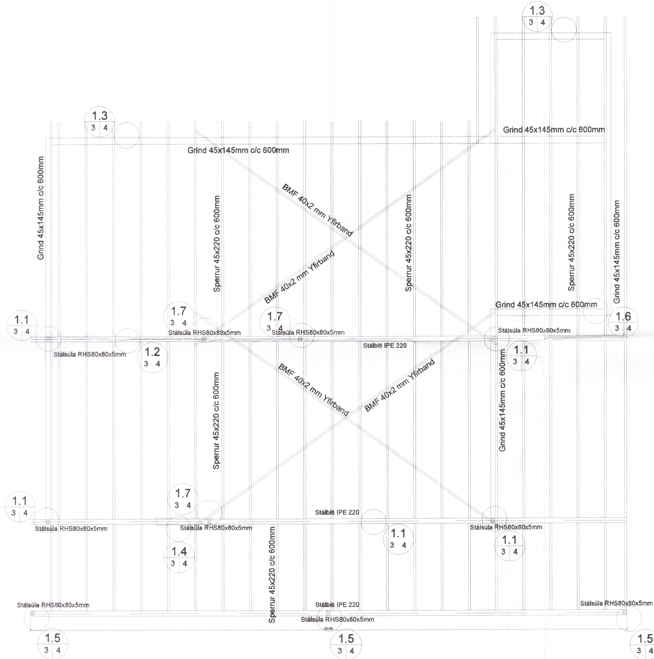
Grunnmynd 1:50
