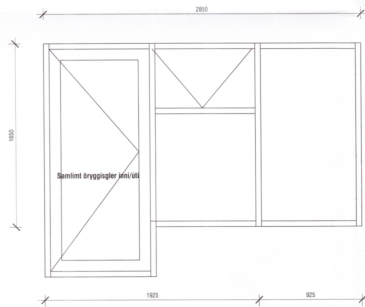
G1 - 1 stk timburgluggi Hurð með paníkíska - neyðarútgangur EN 179
