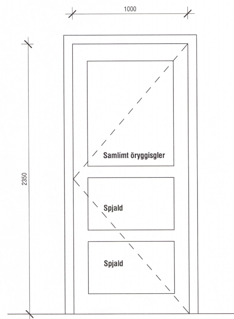
Opnun V-út Neyðaropnun, EN179 handfang Lima efri brún við núverandi hurðir á 1.hæð 25mm álþröskuldur (hjólastólafær)
