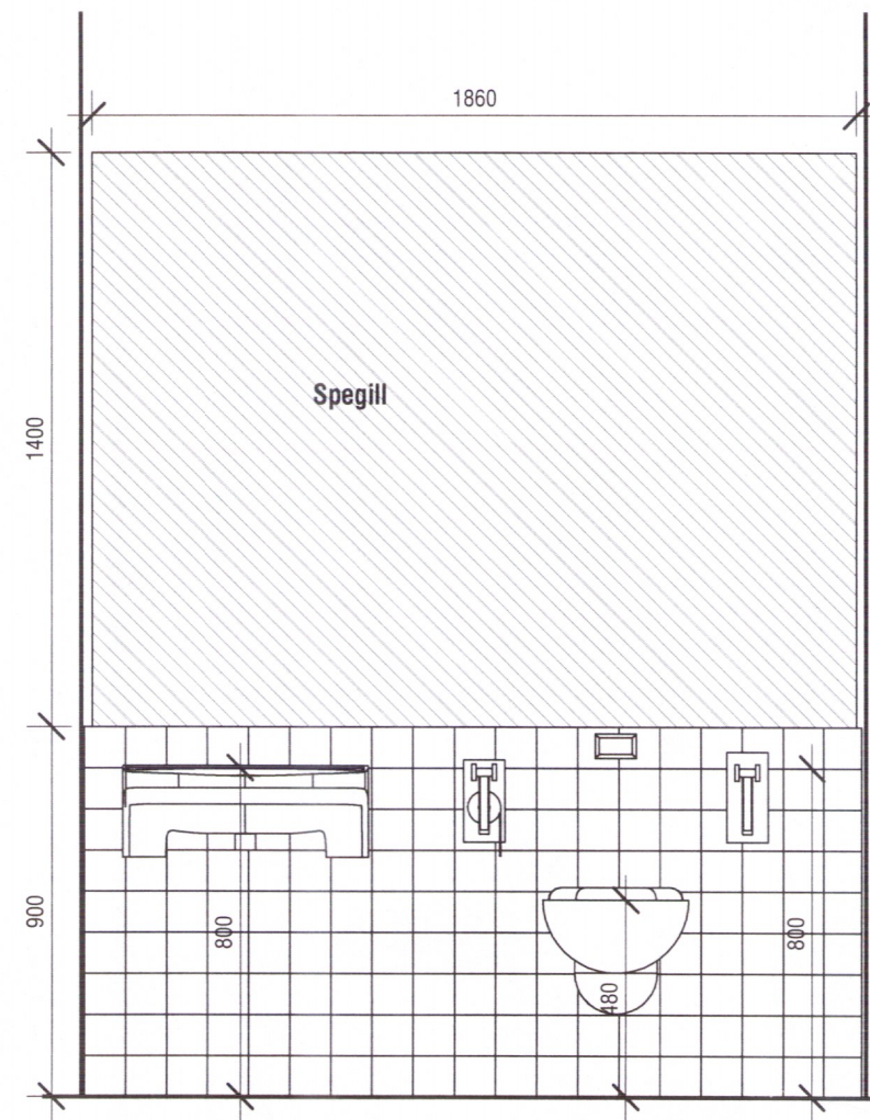
1 Salerni 1 : 20
