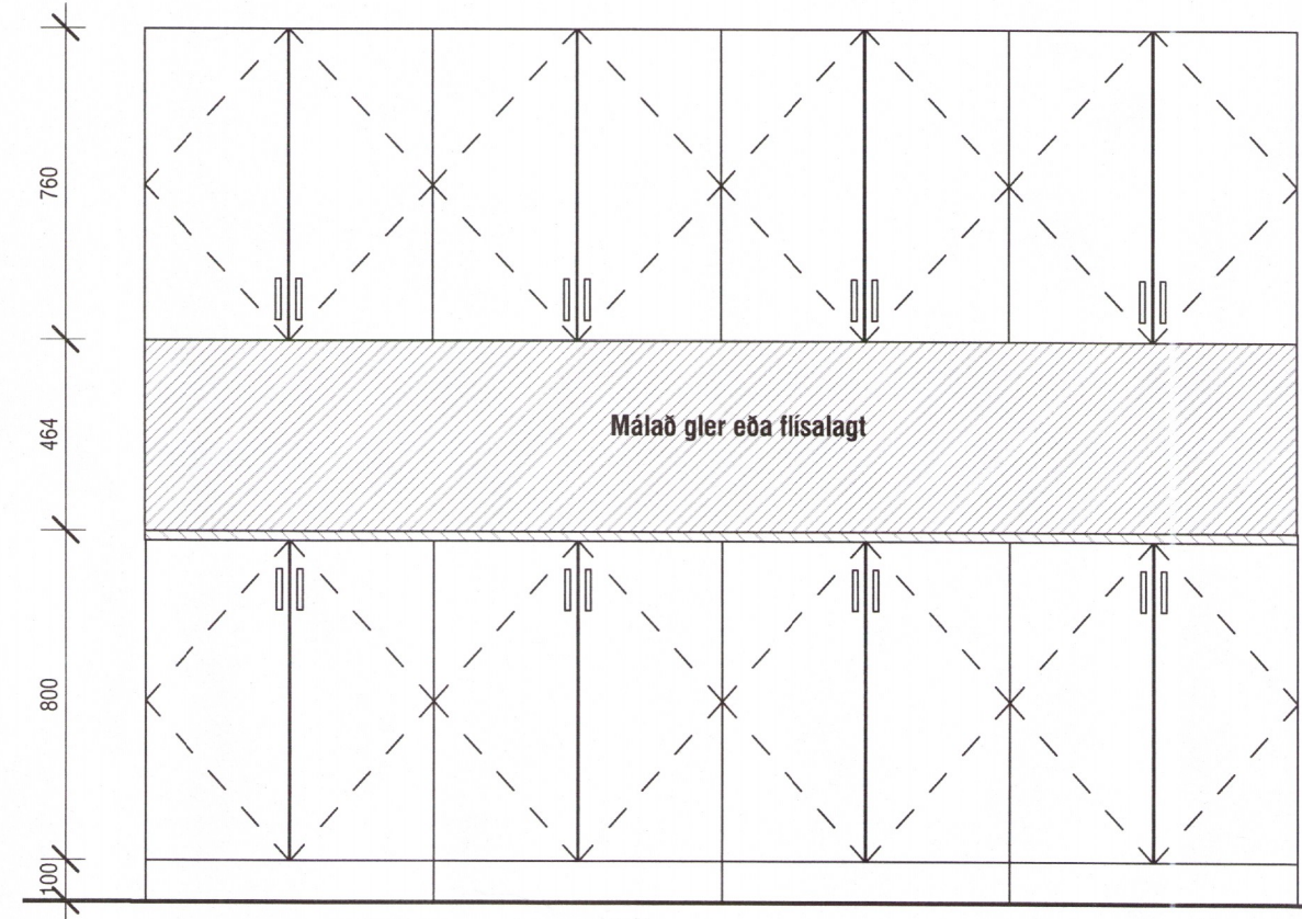
2 Eldhúsinnrétting 1 : 20
