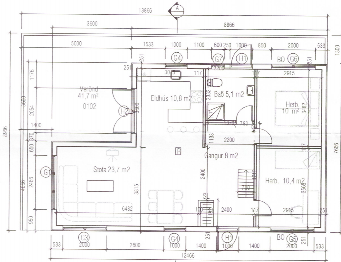
Grunnmynd 1:100
