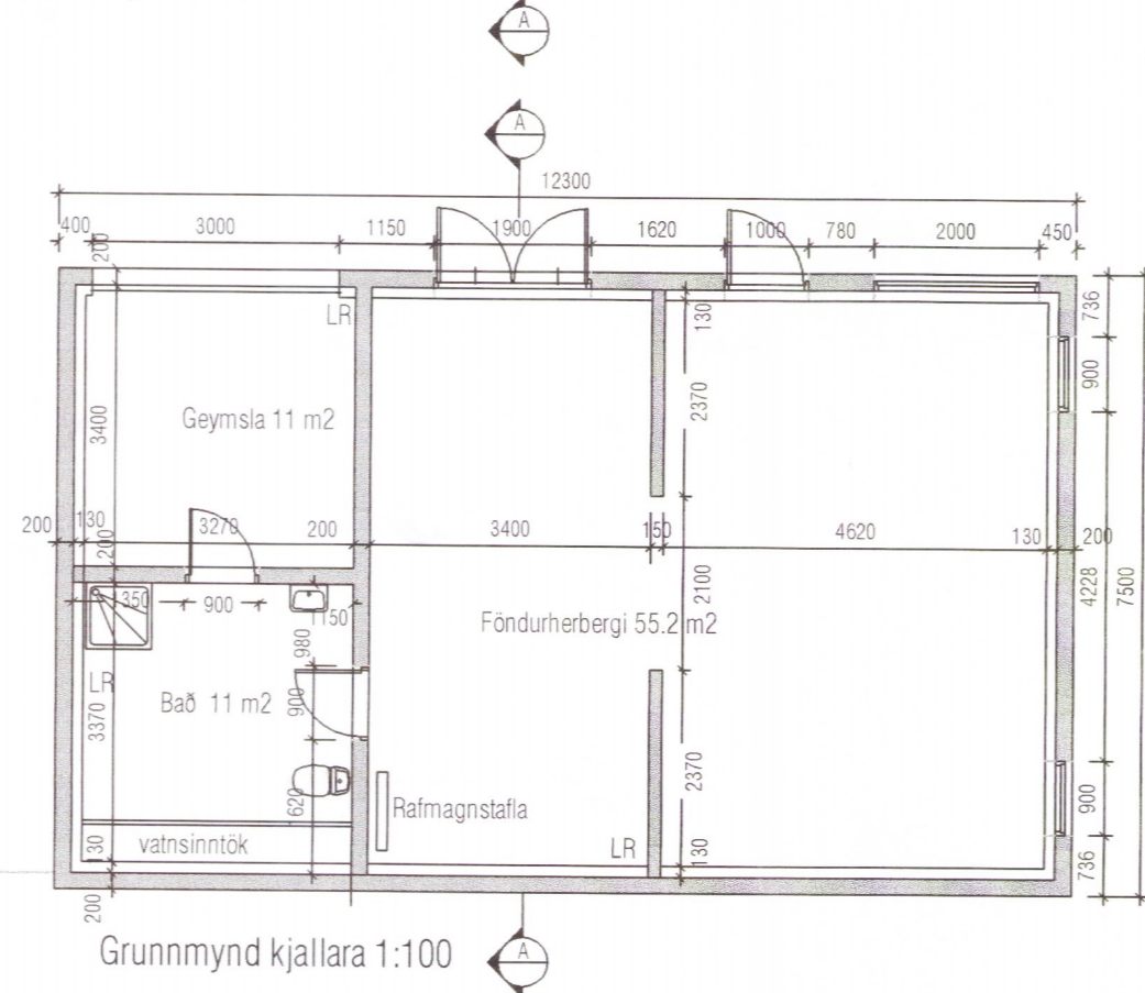
Grunnmynd 1:100
