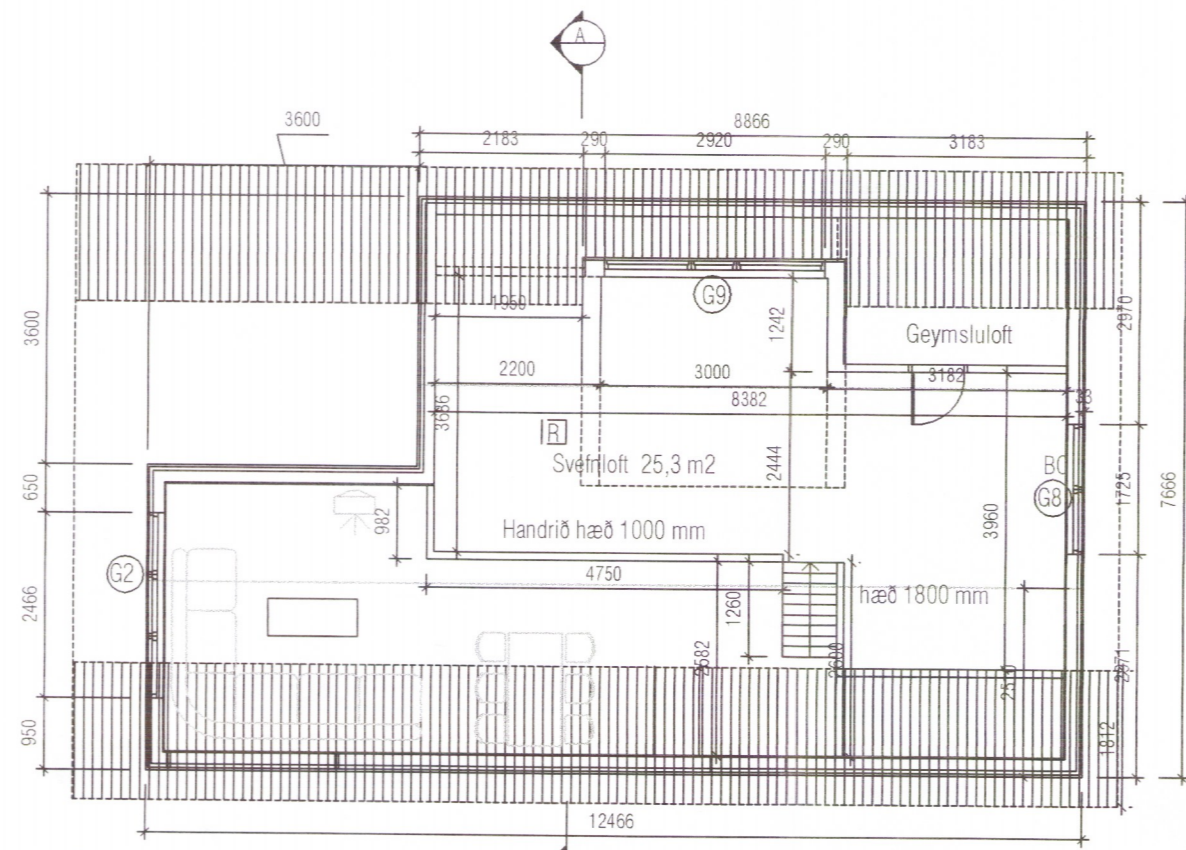
Grunnmynd svefnlofts 1:100
