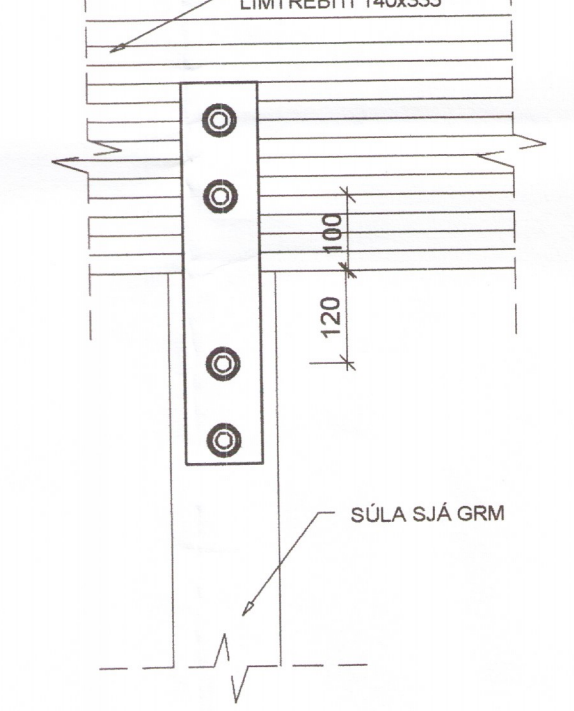
FESTING, F2 1:10
