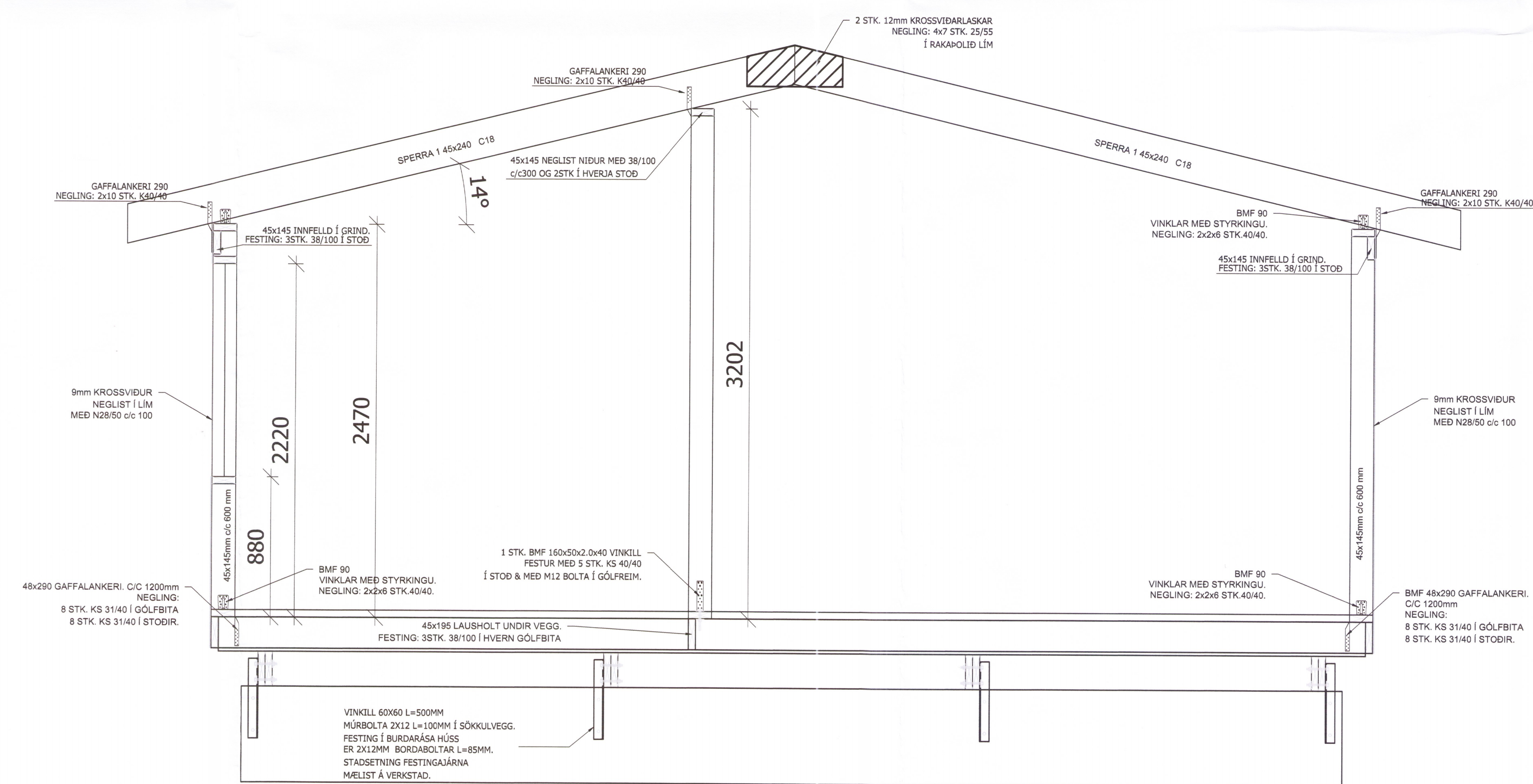
A SNID Í ALRÝMI Mkv 1:20
