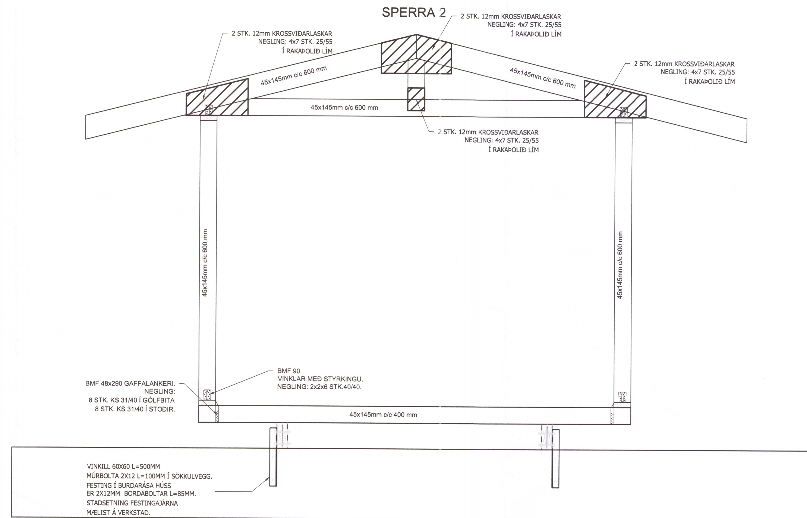
A SNID Í ANDYRI Mkv 1:20
