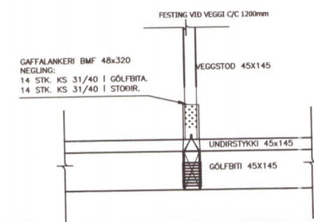
2 FESTINGAR GÓLF VIÐ VEGGI Mkv 1:10
