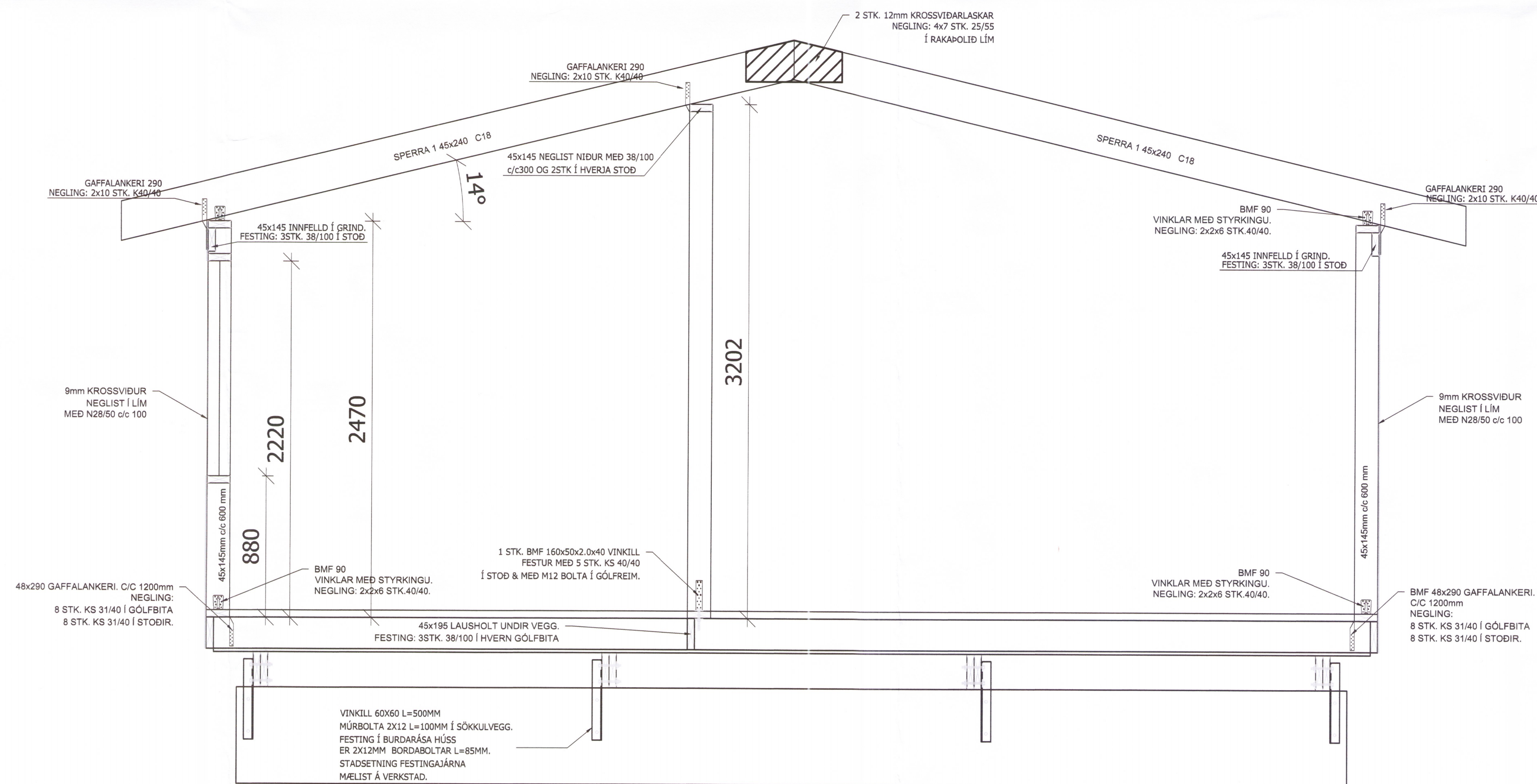
A SNIÐ Í ALRÝMI Mkv 1:20
