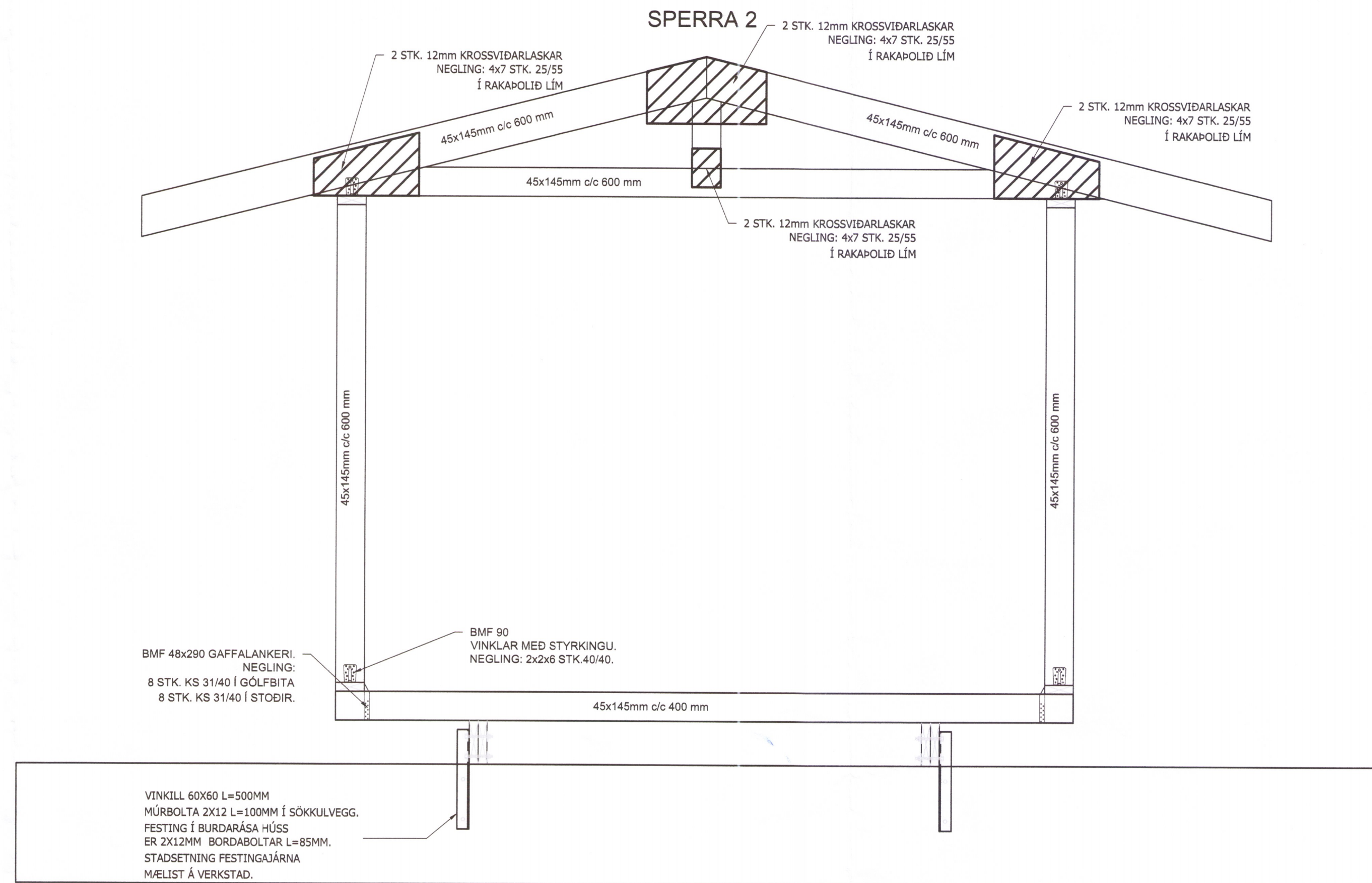
A SNIÐ Í ANDYRI Mkv 1:20
