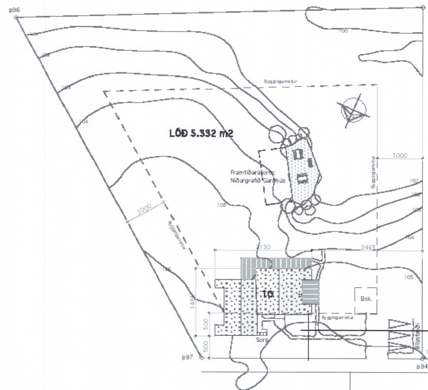
AFSTÖÐUMYND Mkv. 1 : 500
