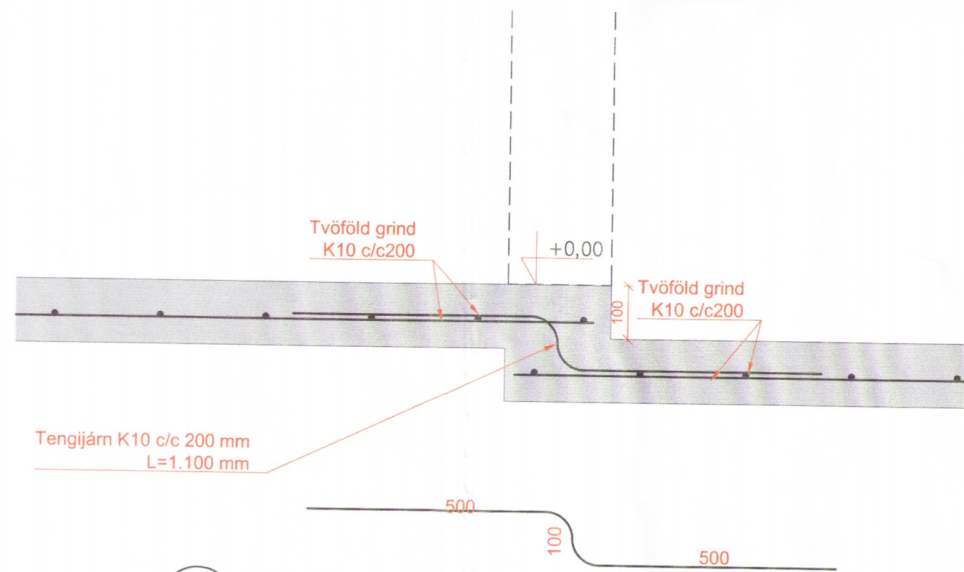
10 Deili 100-01 M 1:10
