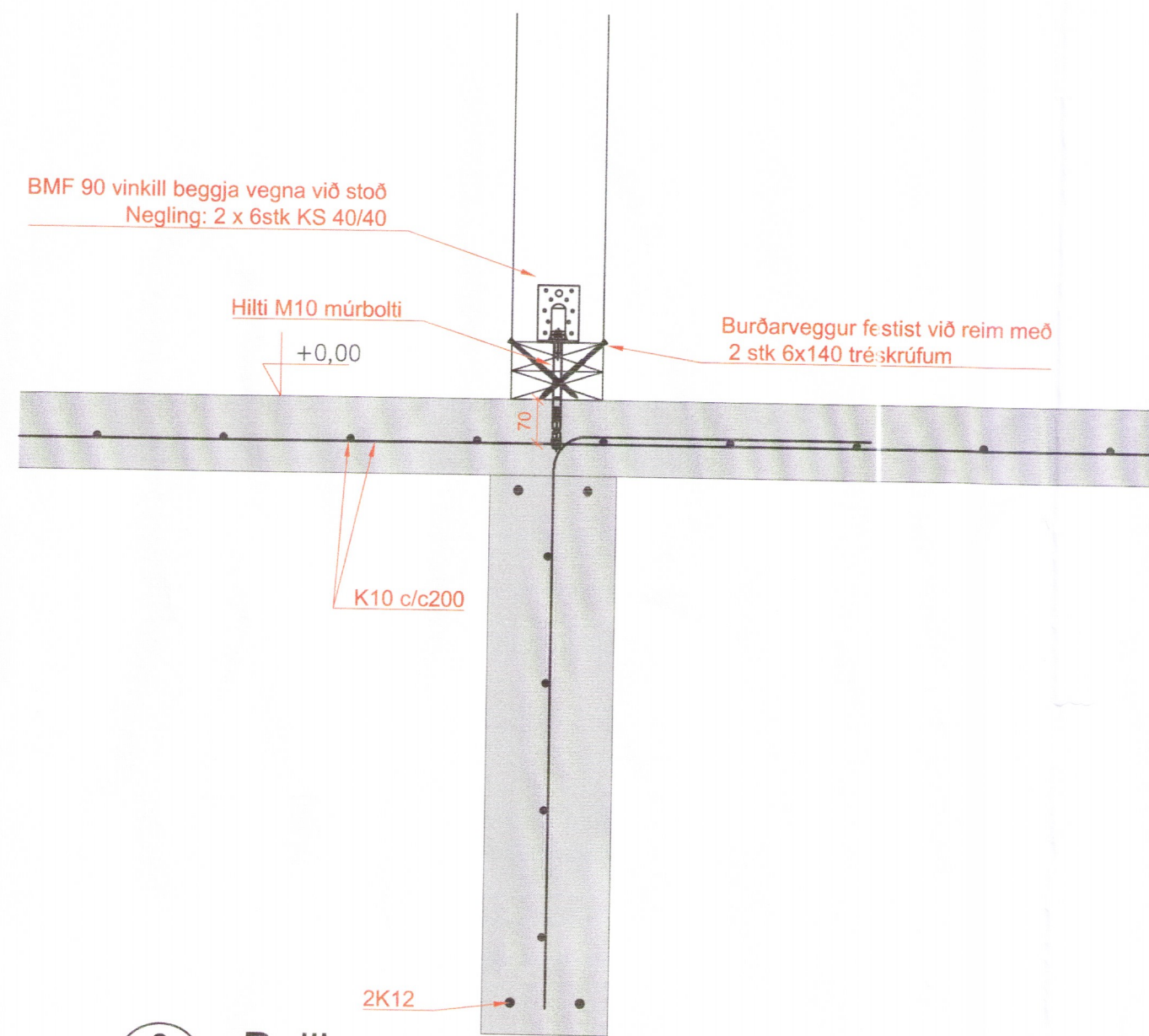
8 Deili 100-01 M 1:10
