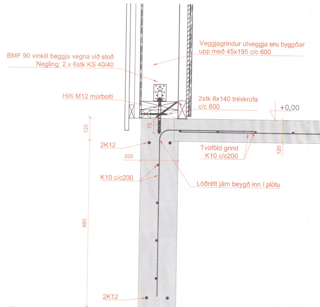
7 Deili 100-01 M 1:10
