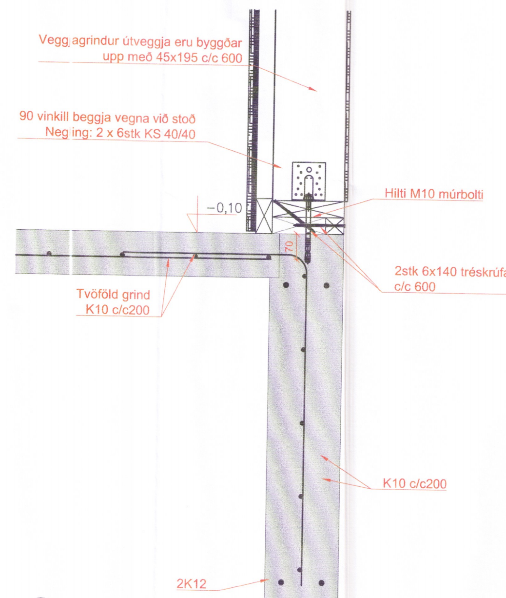
11 Deili 100-01 M 1:10
