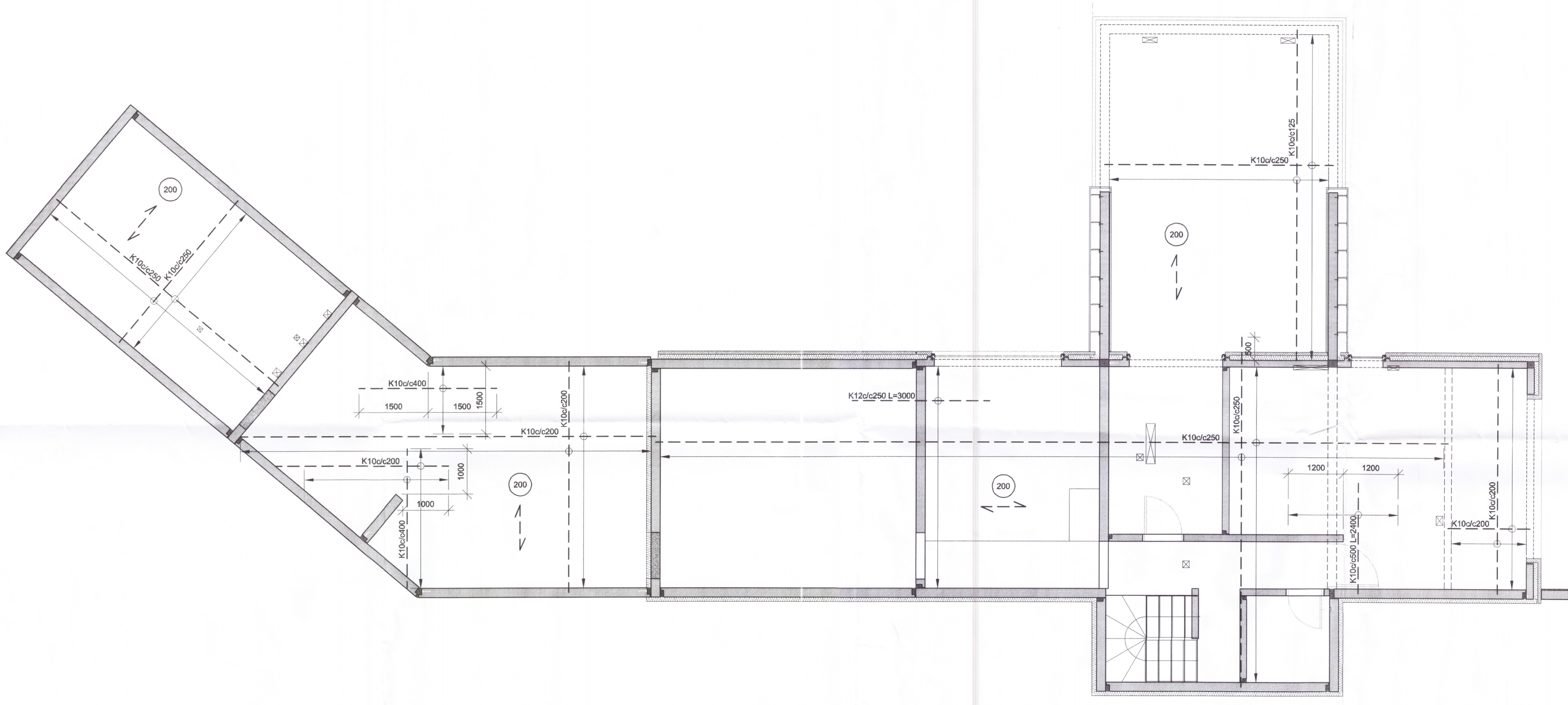
Grunnmynd plötu yfir kjallara, 1:50
