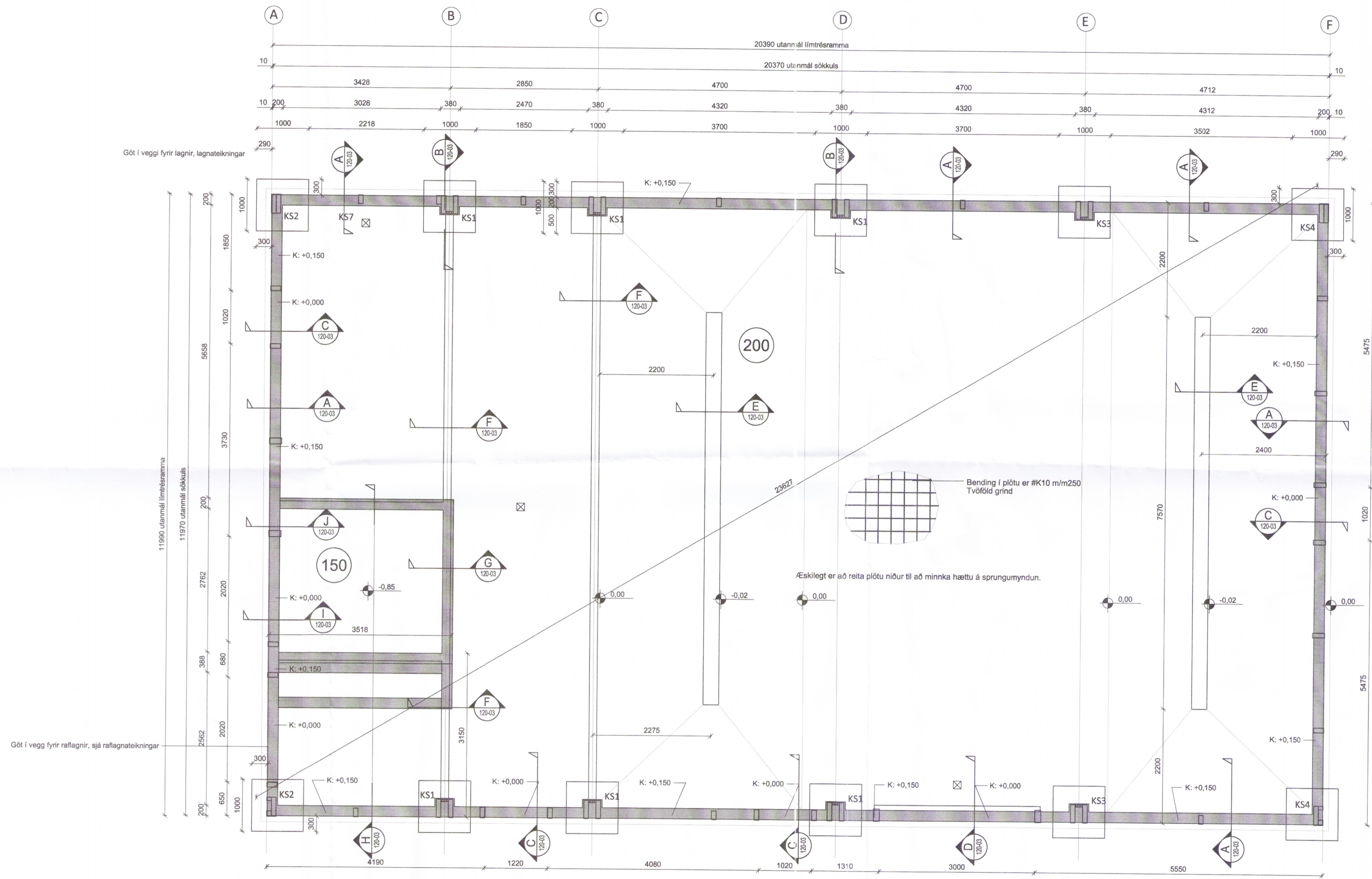
Grunnmynd sökkla og plötu M 1:50
