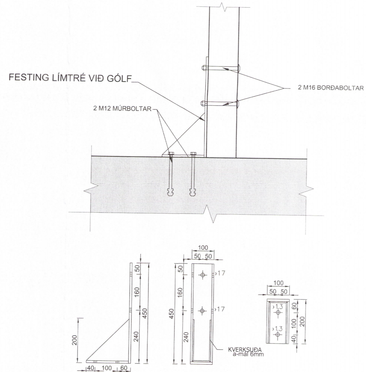
FESTING LÍMTRÉ VIÐ GÓLF MKV. 1:10 UNNIN UR 8mm PÝKKU STÁLI (10 stk.)
