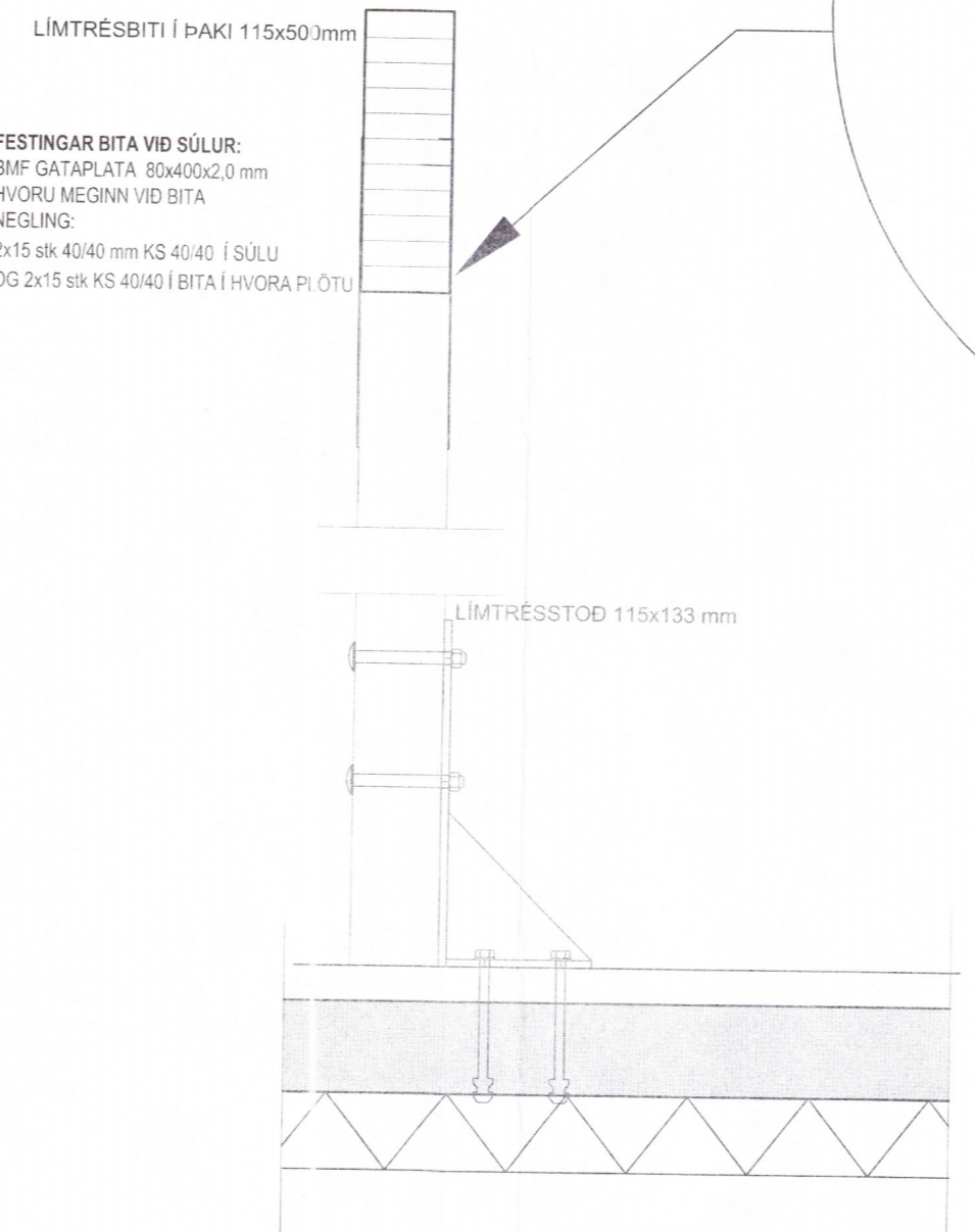
FRÁGANGUR Á LÍMTRÉSBITA OG LÍMTRÉSÚLU VIÐ ÚTVEGGI MKV. 1:10
