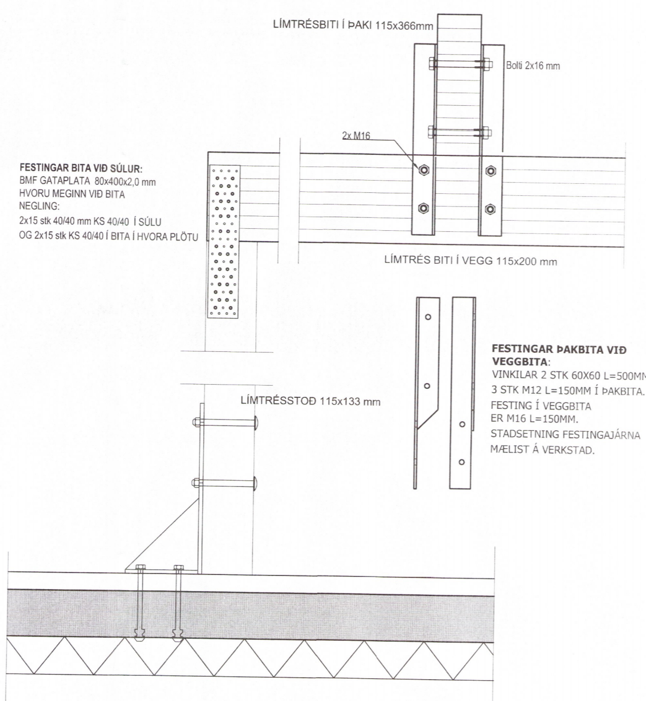
FRÁGANGUR Á LÍMTRÉSBITA VIÐ ÚTVEGGI YFIR GLUGGUM MKV. 1:10
