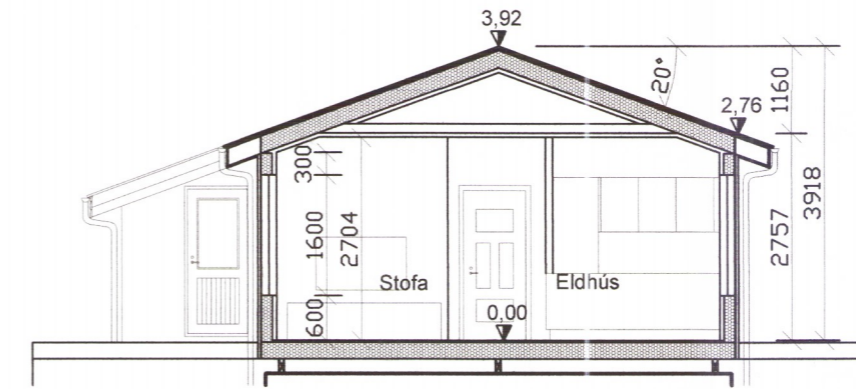
SNID B - 1:100
