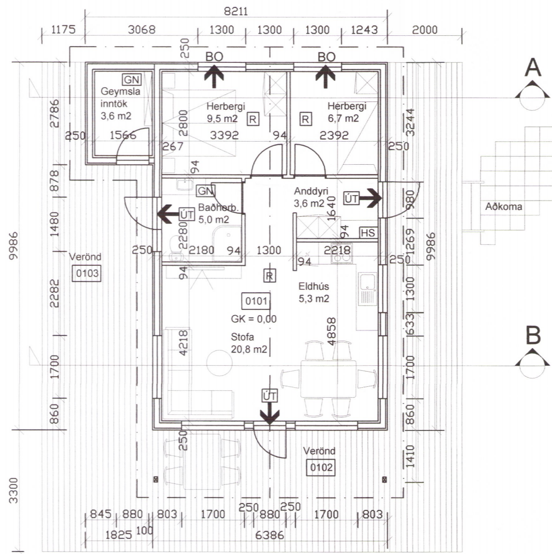
GRUNNMYND - 1:100
