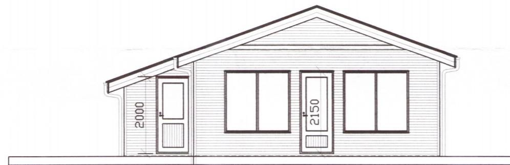
SUDAUSTUR HLIÐ - 1:100
