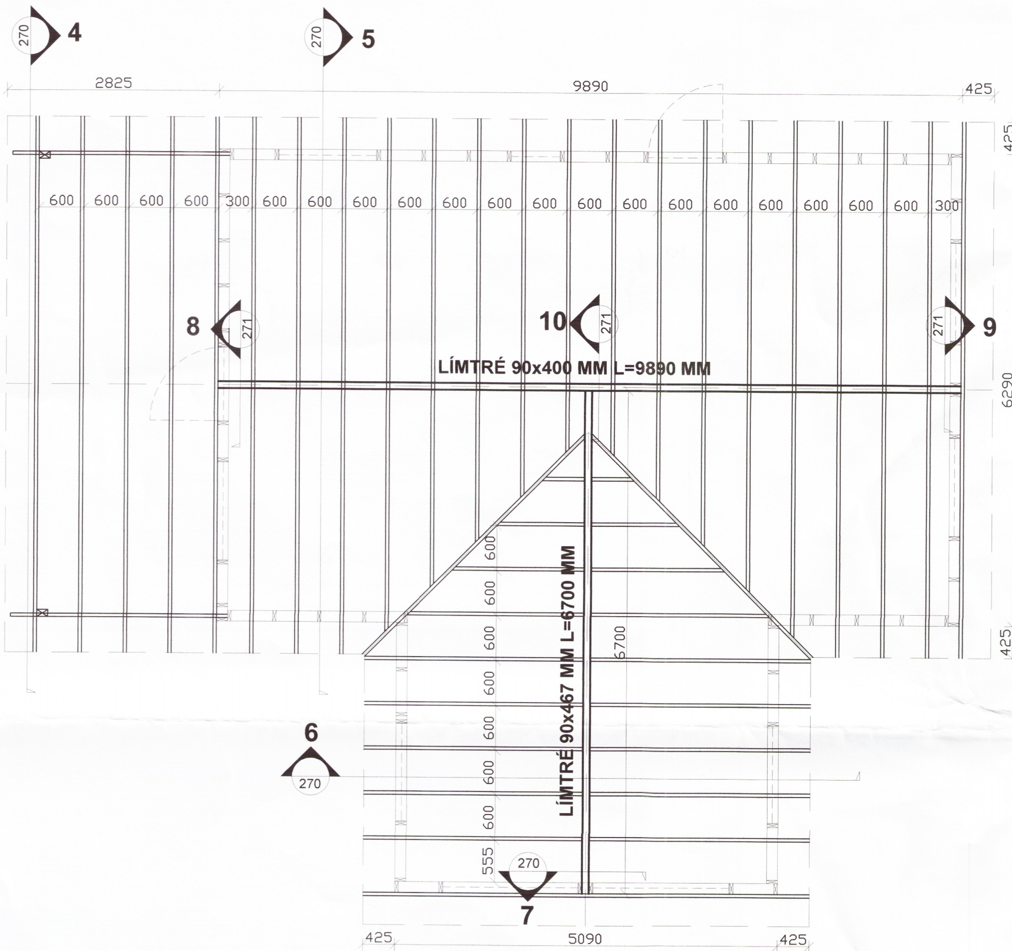
GRUNNMYND - 1:50
