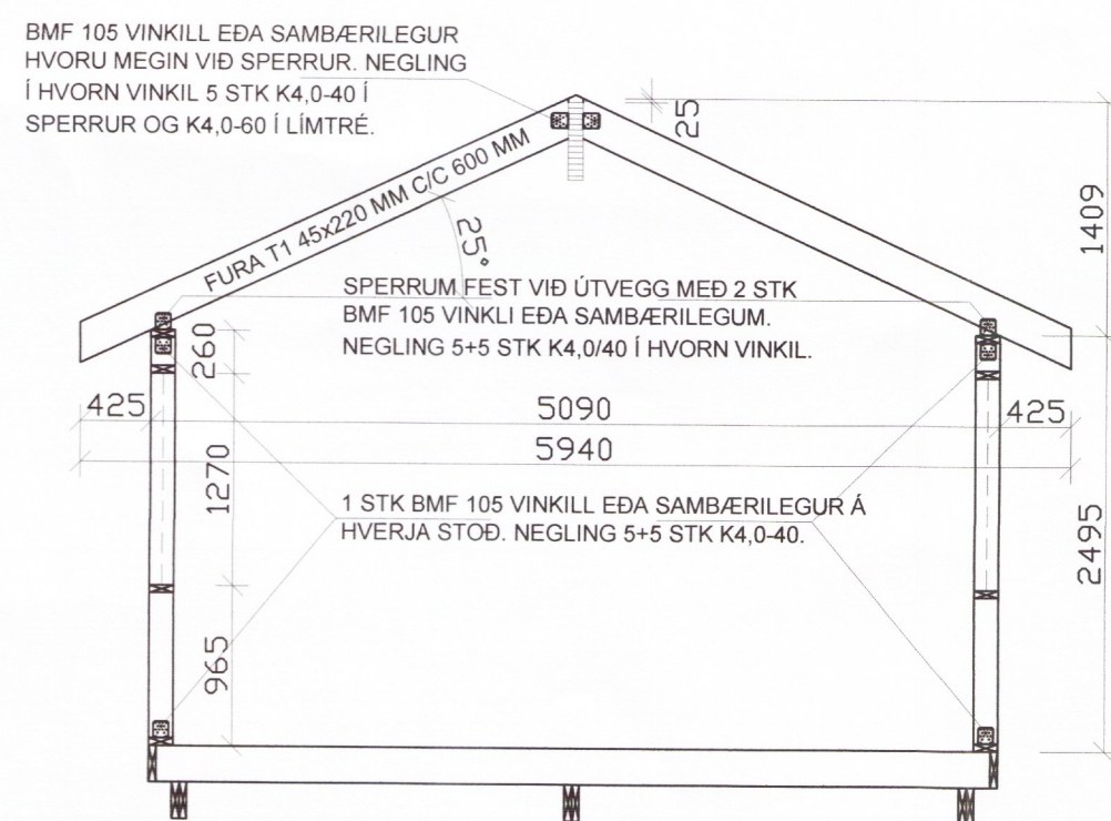
SNID 6 - 1:50
