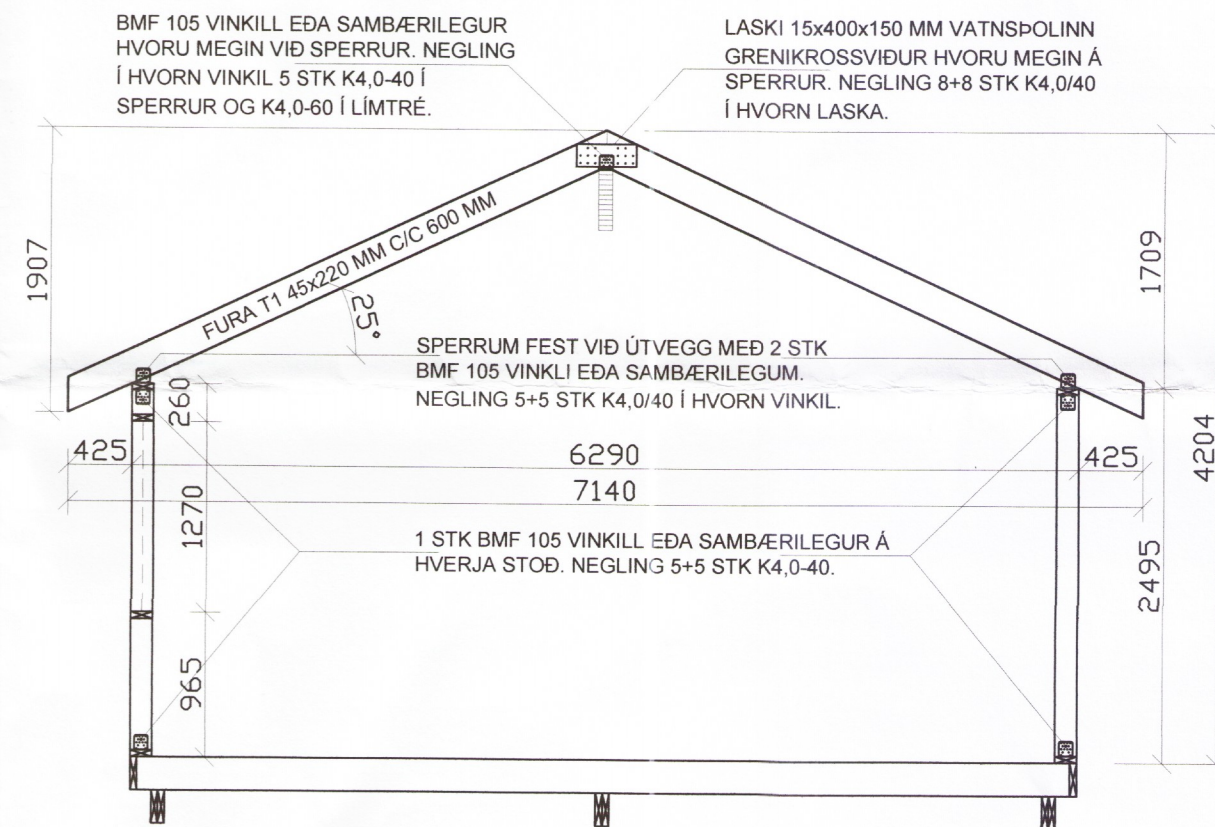
SNID 5 - 1:50
