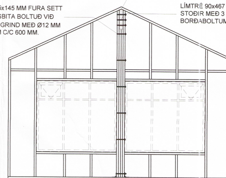
SNID 7 - 1:50
