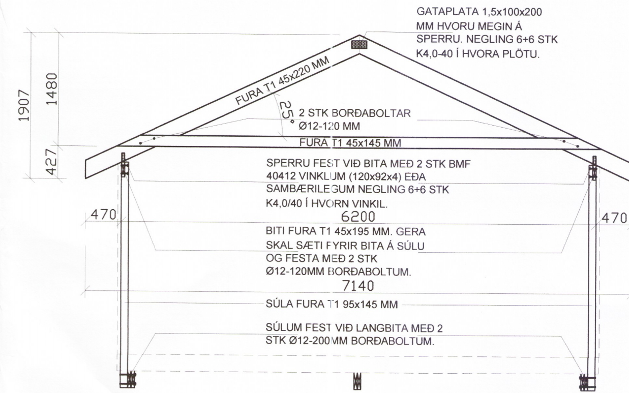
SNID 4 - 1:50
