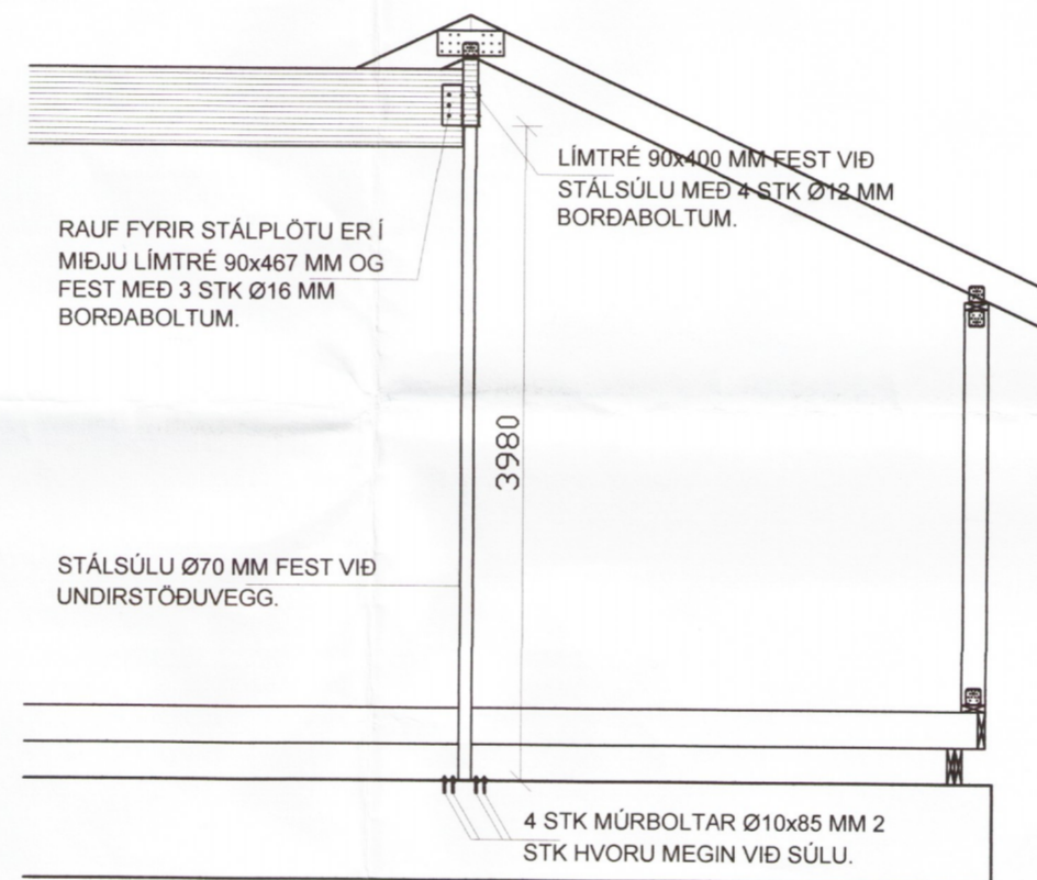
SNIÐ 10 - 1:50
