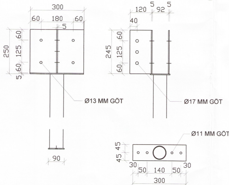
STÁLSÚLA - 1:10
