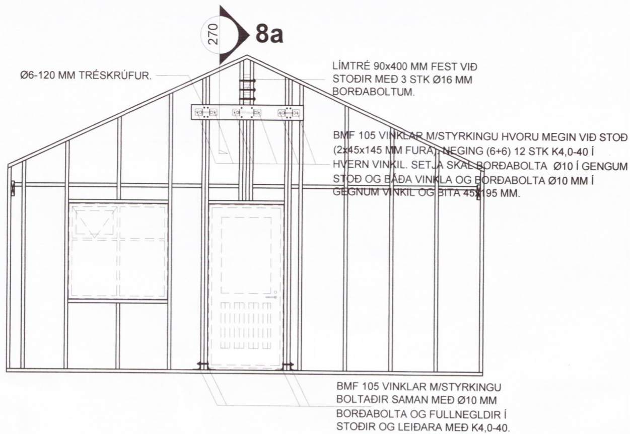
SNIÐ 8 - 1:50
