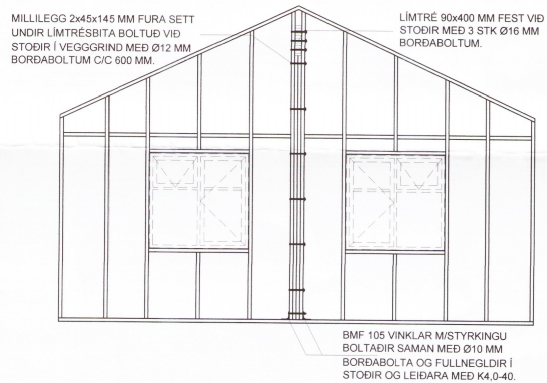
SNIÐ 9 - 1:50
