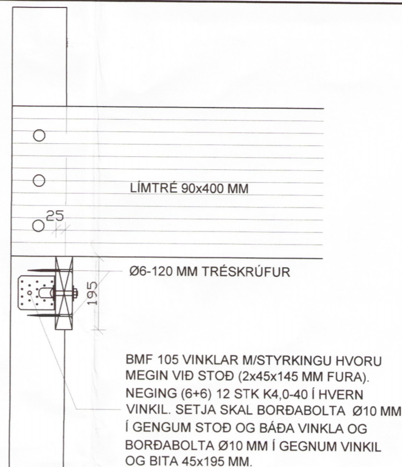
SNIÐ 8a - 1:10
