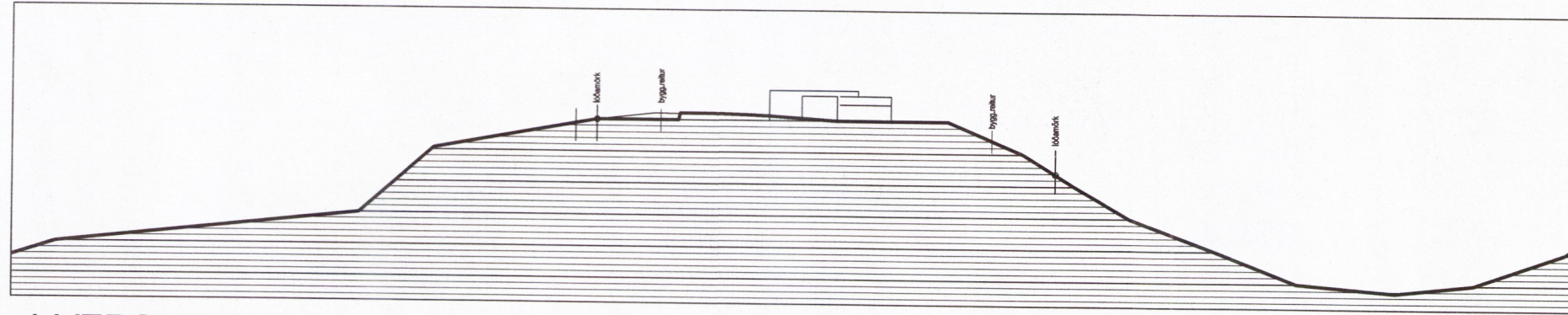
PVERSNIÐ A-A
