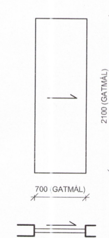
IH-06 1 STK TIMBURHURD, INNIHURD, RENNIHURD LITUR INNI: VELJIST Í SAMRÁÐI VÍÐ ARKITEKT LITUR ÚTI: VELJIST Í SAMRÁÐI VÍÐ ARKITEKT
