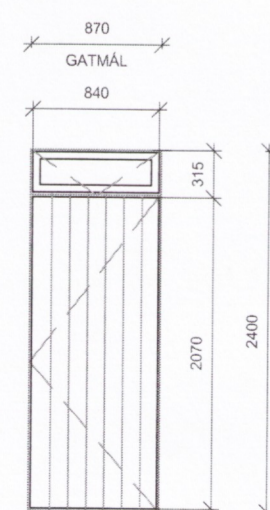
UH-05 1 STK TIMBURHURD, KLÆDD MÈÐ LERKI LITUR INNI: VELJIST Í SAMRÁÐI VÍÐ ARKITEKT LITUR ÚTI: ÓMÈDHONÐLAÐ LERKI
