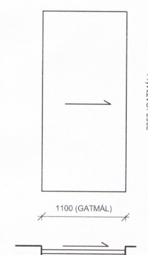
IH-04 2 STK TIMBURHURD, INNIHURD, RENNIHURD LITUR INNI: VELJIST Í SAMRÁÐI VÍÐ ARKITEKT LITUR ÚTI: VELJIST Í SAMRÁÐI VÍÐ ARKITEKT
