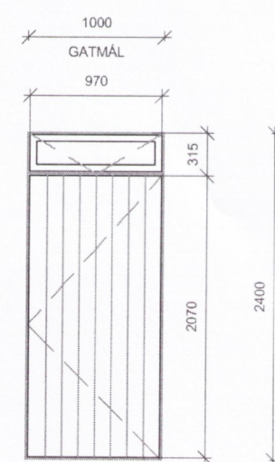
UH-06 1 STK TIMBURHURD, KLÆDD MÈÐ LERKI LITUR INNI: VELJIST Í SAMRÁÐI VÍÐ ARKITEKT LITUR ÚTI: ÓMÈDHONÐLAÐ LERKI
