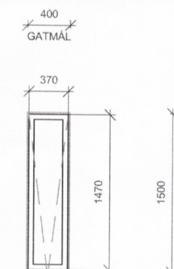
G-06 1 STK ÁLTIMBURGLUGGI LITUR INNI: VELJIST Í SAMRÁÐI VÍÐ ARKITEKT LITUR ÚTI: SVARTUR
