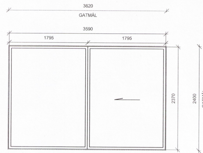
UH-02 2 STK SAMTALS ÁLTIMBUR RENNIHURD LITUR INNI: VELJIST Í SAMRÁÐI VÍÐ ARKITEKT LITUR ÚTI: SVARTUR
