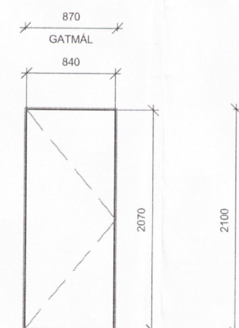
IH-02 1 STK TIMBURHURD, INNIHURD LITUR INNI: VELJIST Í SAMRÁÐI VÍÐ ARKITEKT LITUR ÚTI: VELJIST Í SAMRÁÐI VÍÐ ARKITEKT
