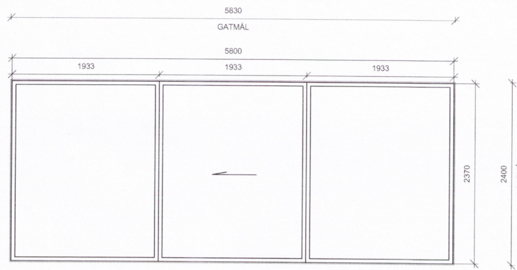
UH-01 1 STK SAMTALS ÁLTIMBUR RENNIHURD, LOFTUNARRIST Í PROFÍLUM LITUR INNI: VELJIST Í SAMRÁÐI VÍÐ ARKITEKT LITUR ÚTI: SVARTUR
