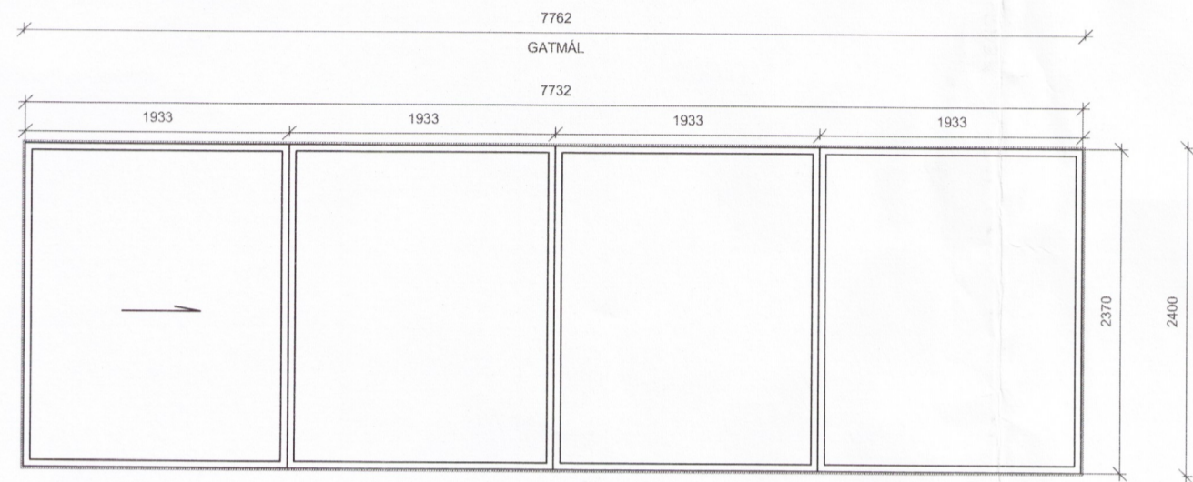
UH-03 1 STK SAMTALS ÁLTIMBUR RENNIHURD, LOFTUNARRIST Í PROFÍLUM LITUR INNI: VELJIST Í SAMRÁÐI VÍÐ ARKITEKT LITUR ÚTI: SVARTUR
