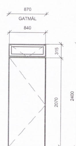
UH-09 1 STK ÁLTIMBURHURD LITUR INNI: VELJIST Í SAMRÁÐI VÍÐ ARKITEKT LITUR ÚTI: SVARTUR
