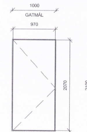
UH-07 1 STK ÁLTIMBURHURD LITUR INNI: VELJIST Í SAMRÁÐI VÍÐ ARKITEKT LITUR ÚTI: SVARTUR
