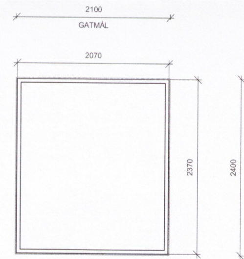
G-02 1 STK ÁLTIMBURGLUGGI LITUR INNI: VELJIST Í SAMRÁÐI VÍÐ ARKITEKT LITUR ÚTI: SVARTUR
