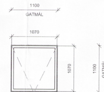
G-05 1 STK ÁLTIMBURGLUGGI LITUR INNI: VELJIST Í SAMRÁÐI VÍÐ ARKITEKT LITUR ÚTI: SVARTUR
