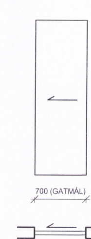
IH-05 1 STK TIMBURHURD, INNIHURD, RENNIHURD LITUR INNI: VELJIST Í SAMRÁÐI VÍÐ ARKITEKT LITUR ÚTI: VELJIST Í SAMRÁÐI VÍÐ ARKITEKT
