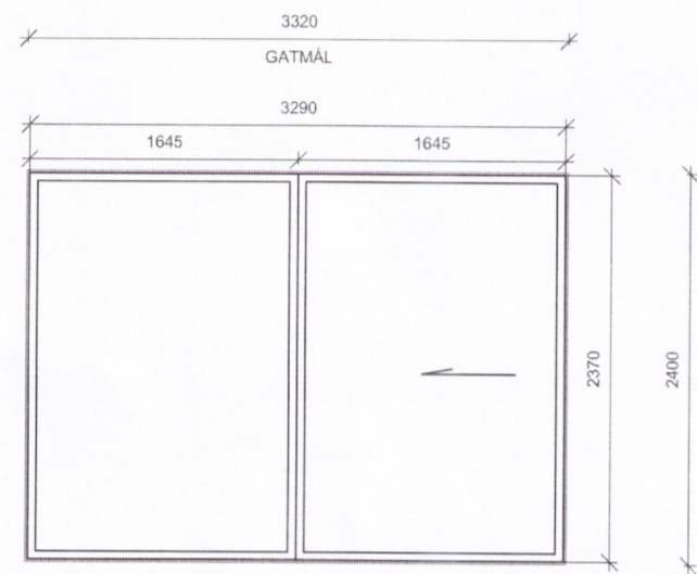
UH-04 1 STK SAMTALS ÁLTIMBUR RENNIHURD LITUR INNI: VELJIST Í SAMRÁÐI VÍÐ ARKITEKT LITUR ÚTI: SVARTUR
