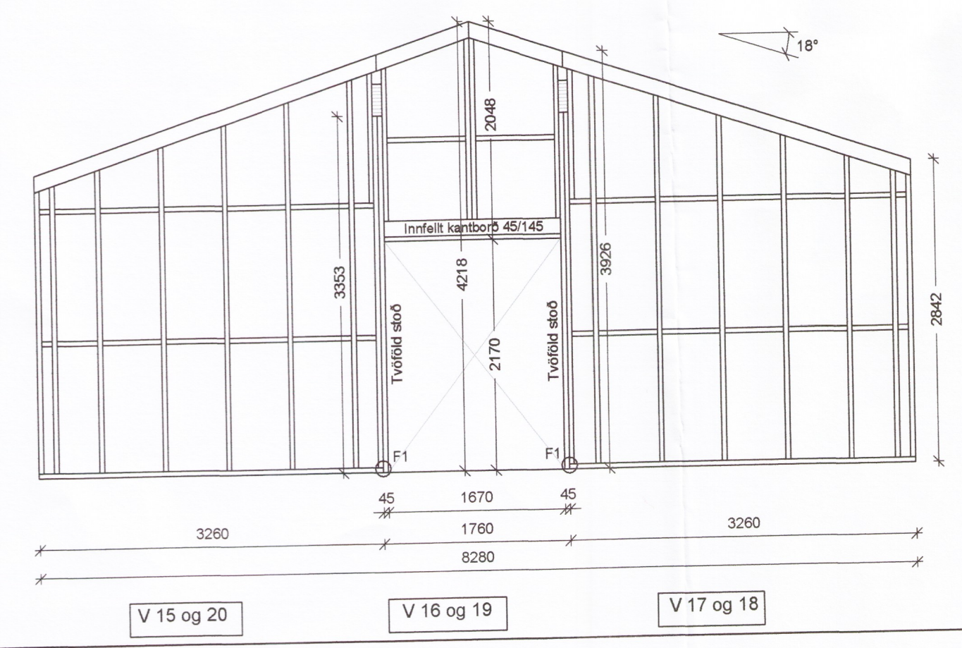
ÁSYND VEGGJAGRINDA MKV. 1:50
