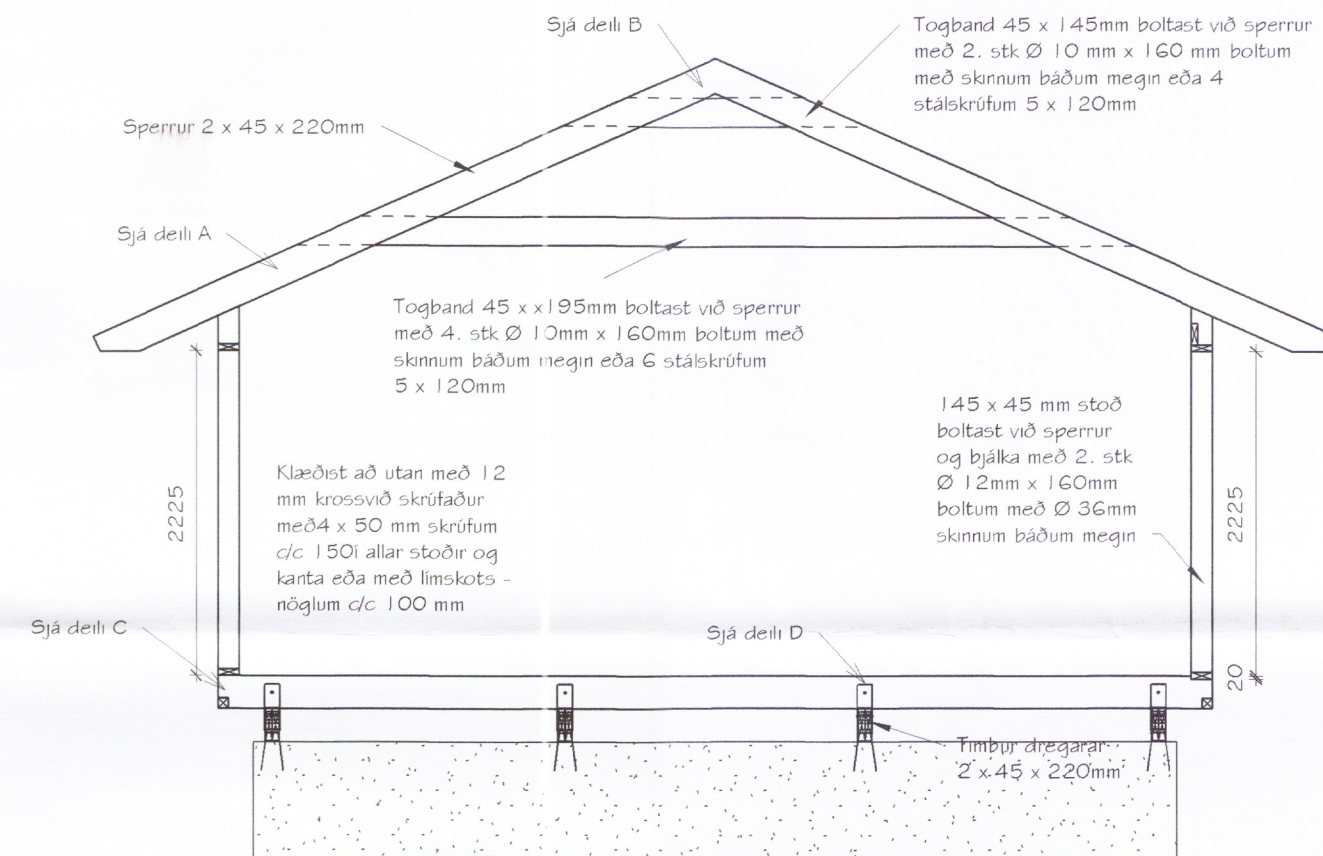
Snið A - A 1 : 50
