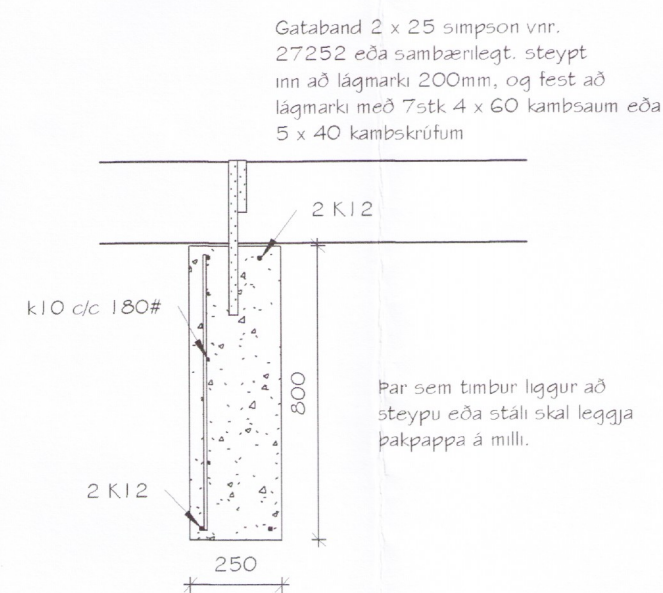
Deili A. 1 : 20
