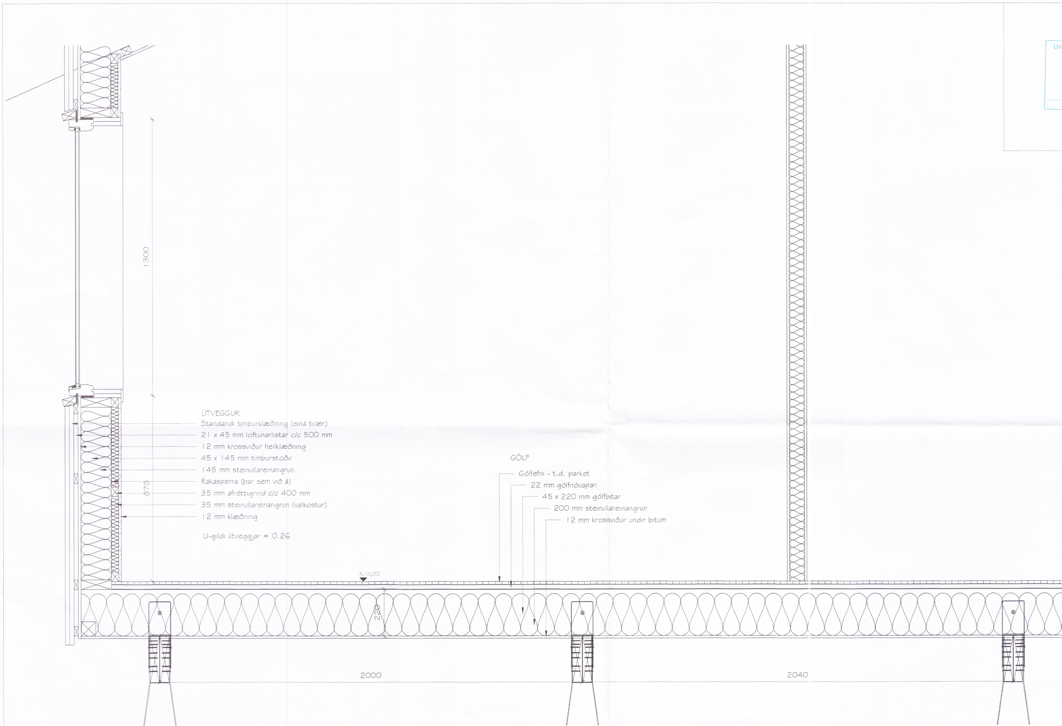
Deiliteikning B 1 : 10
