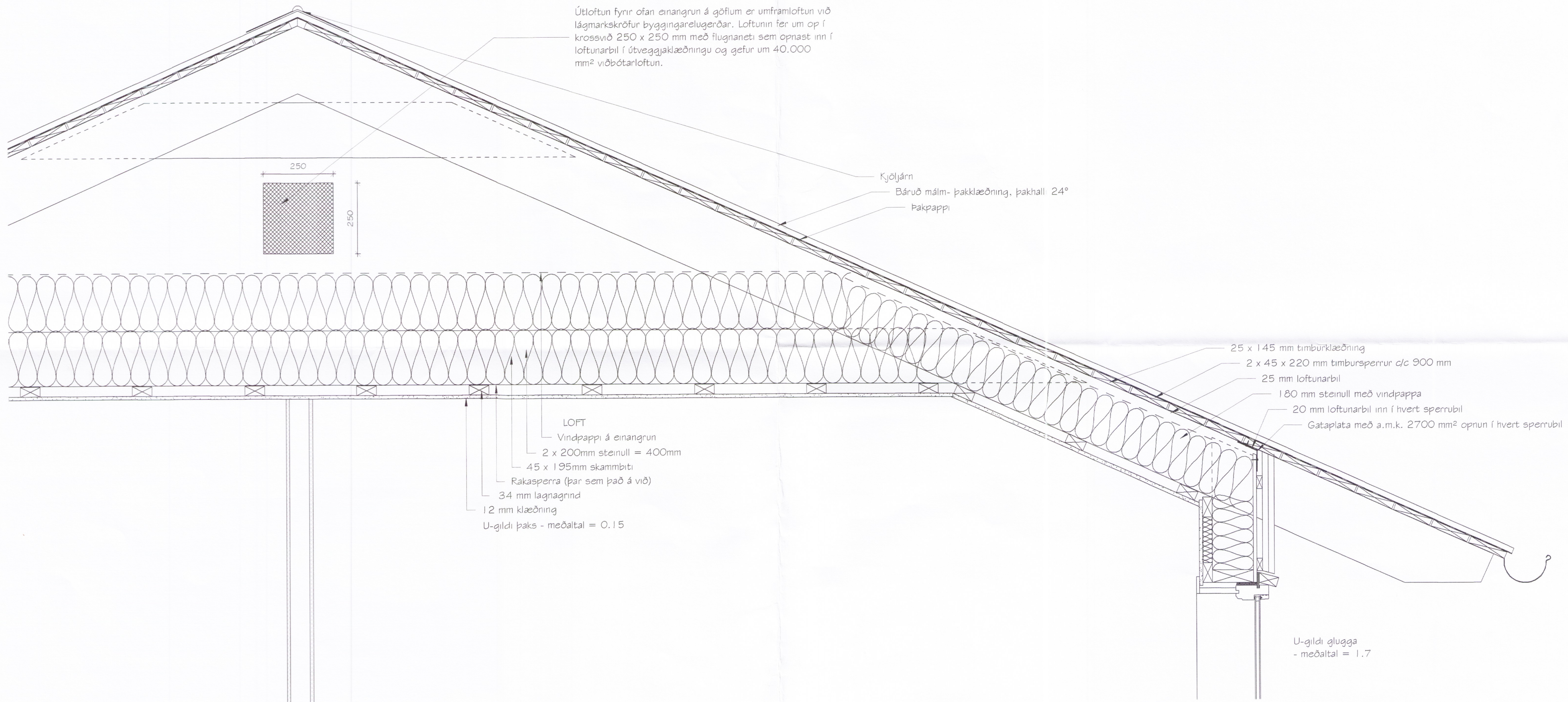
Deiliteikning A 1 : 10
