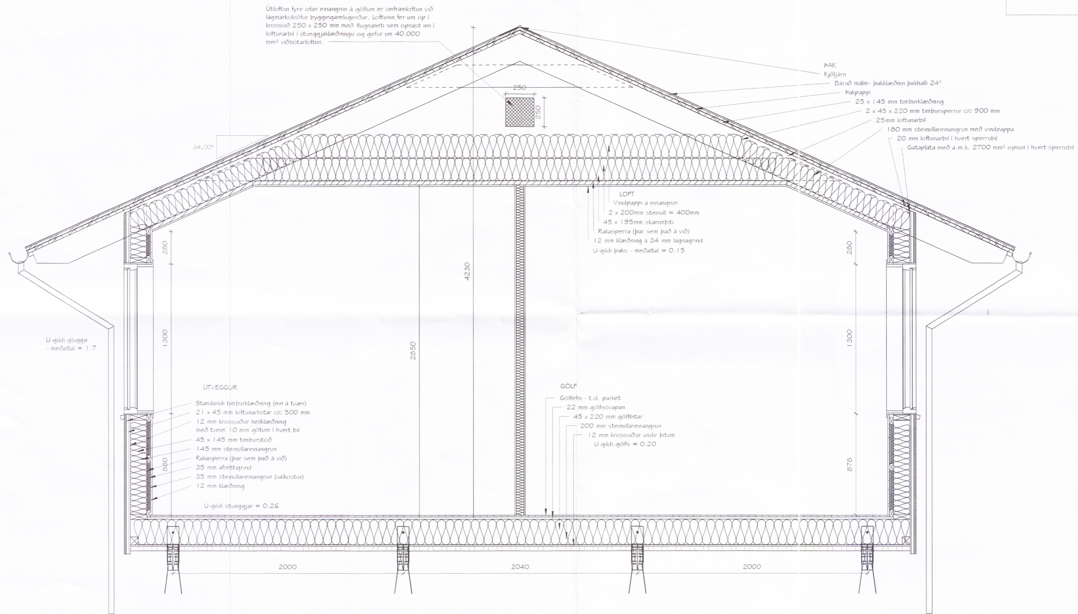
Snið A-A . 1 : 20
