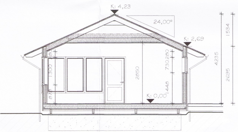
Snið A-A 1 : 100
