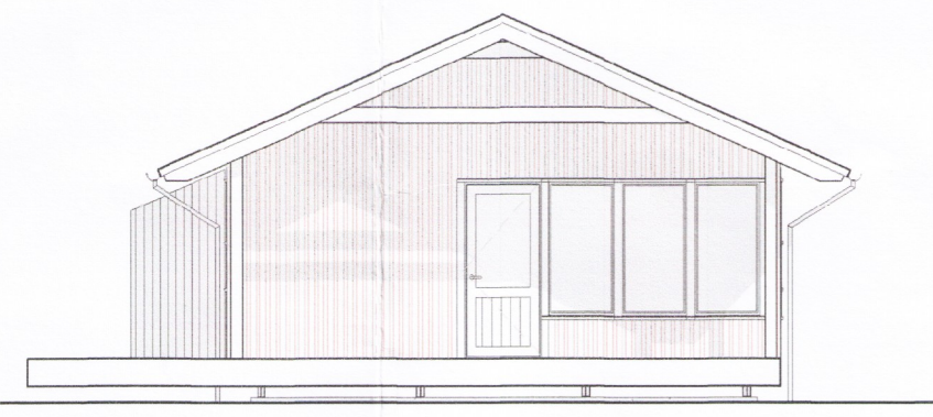
Suðurgafi 1 : 100
