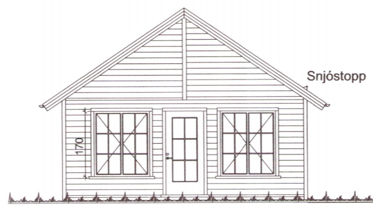
Vesturhlið 1:100
