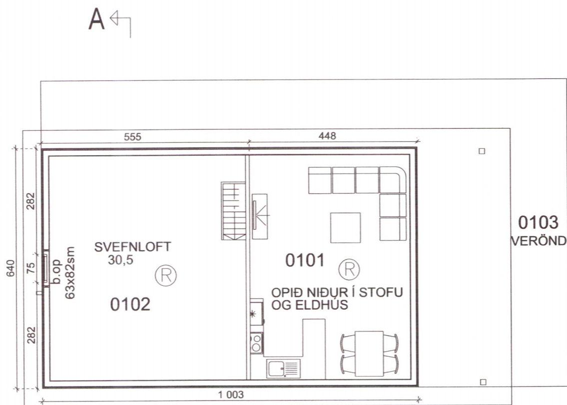
Svefnloft Grunnmynd 1:100
