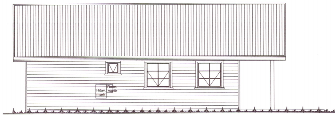
Norðurhlið 1:100
