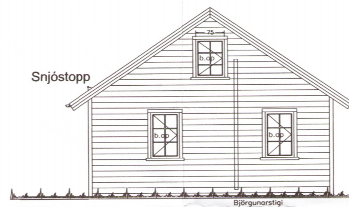
Austurhlið 1:100
