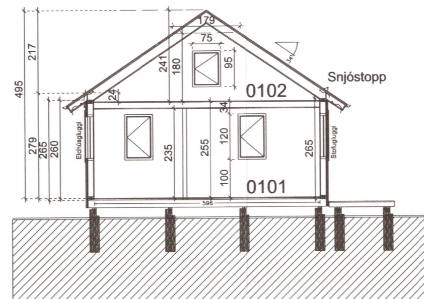
Snið A-A 1:100
