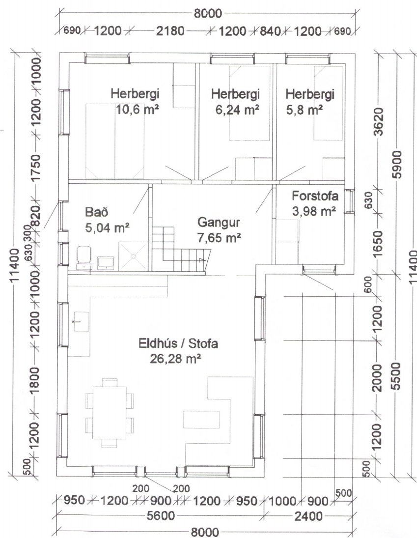
Grunnmynd fyrir breytingu
