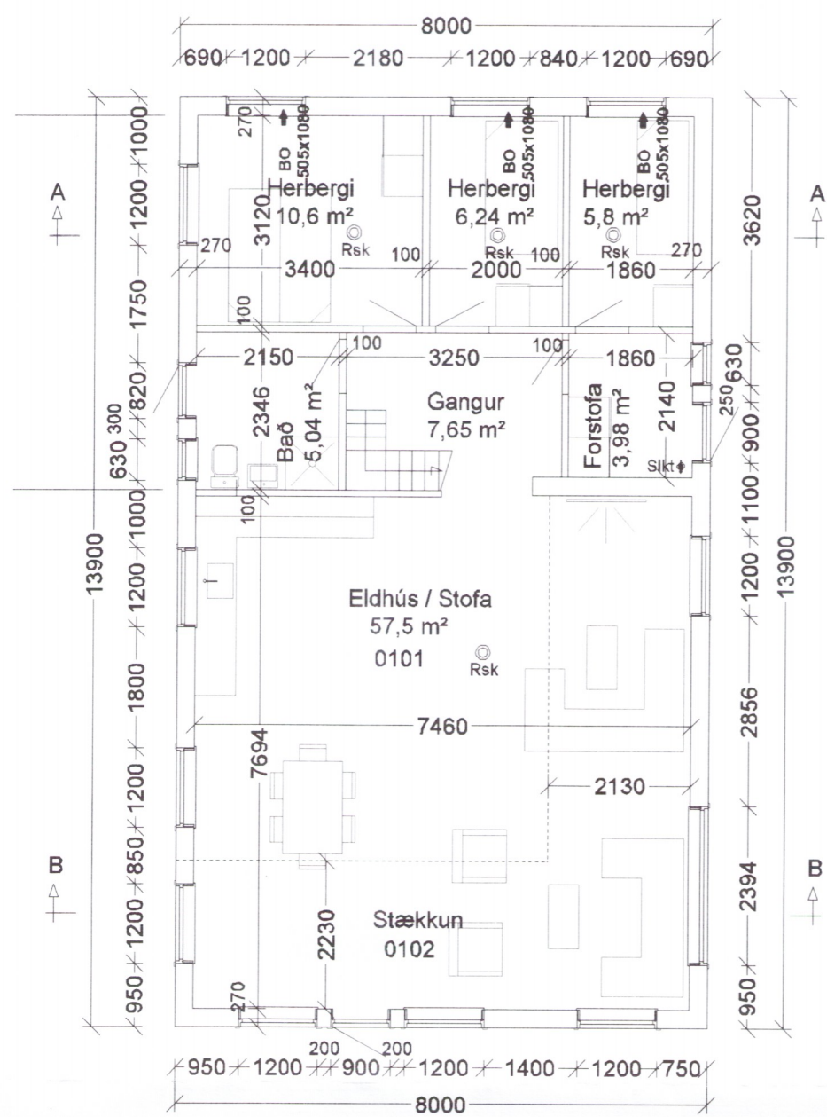
Grunnmynd eftir breytingu
