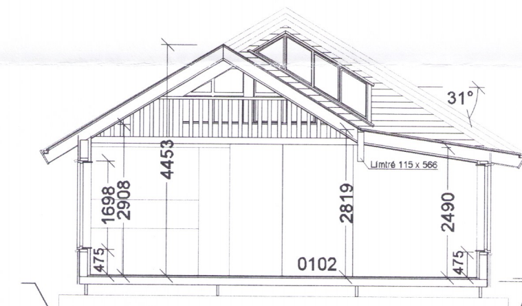
Snið B - B
