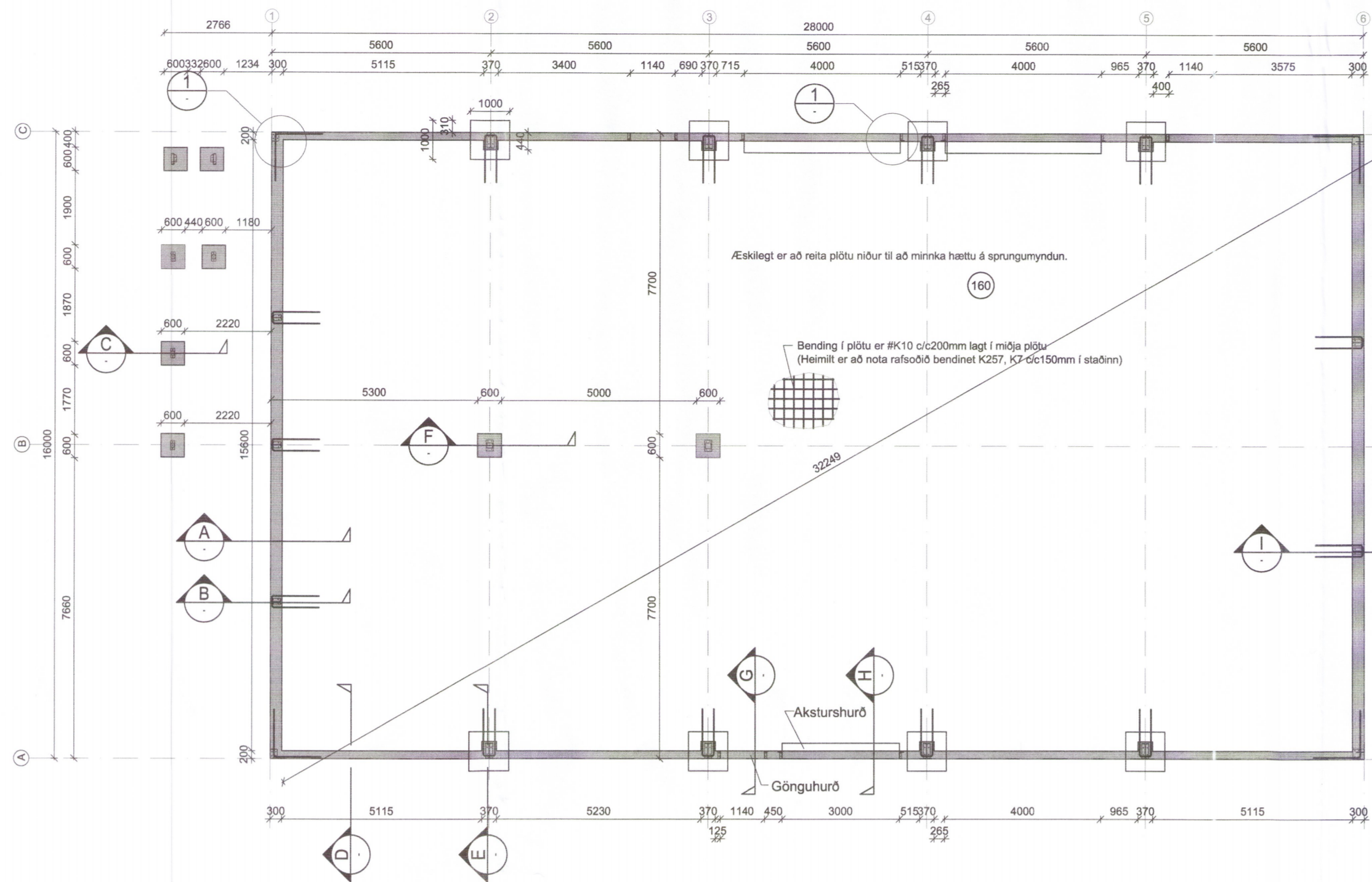
Grunnmynd jarðhæðar M 1:100
