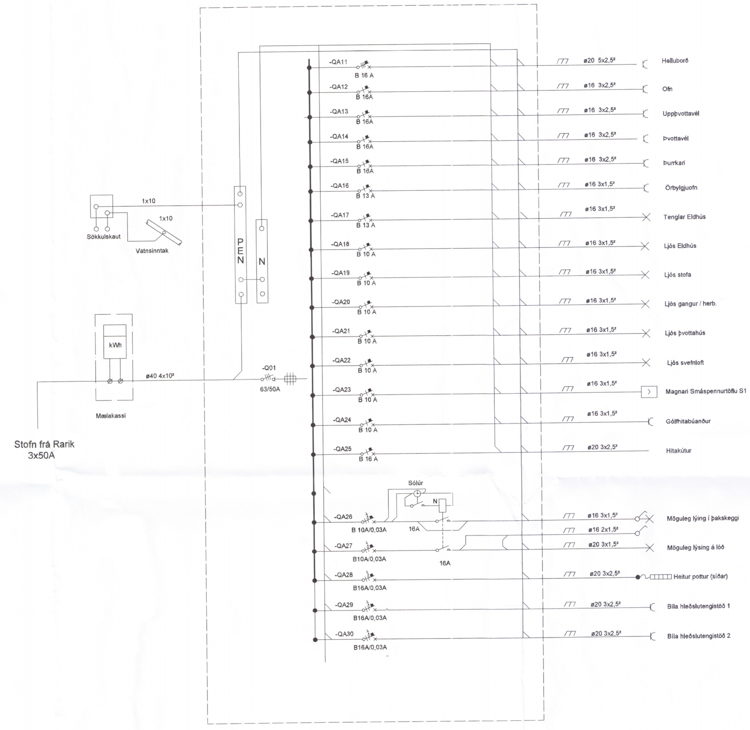
TAFLA -A1 Aðaltafla EINLÍNUMYND
