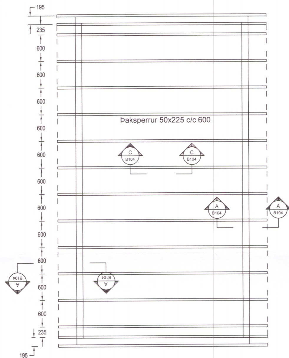
Grunnmynd 1:50
