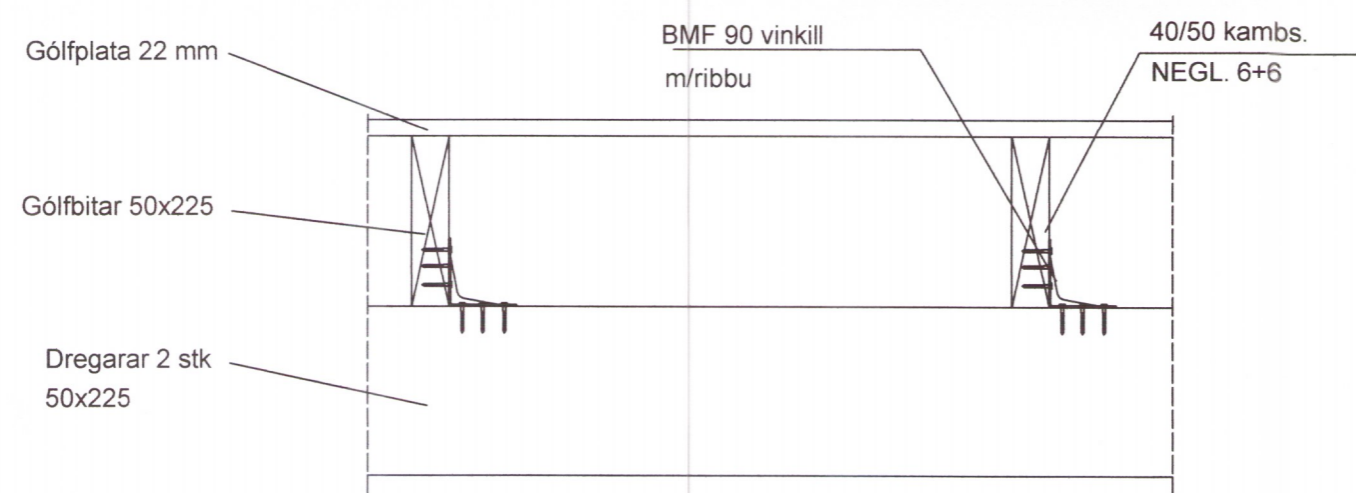
Festing dregarar/gólfbitar 1:10
