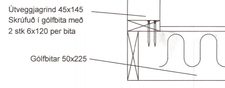
Vegggrindur/gólfbitar 1:10
