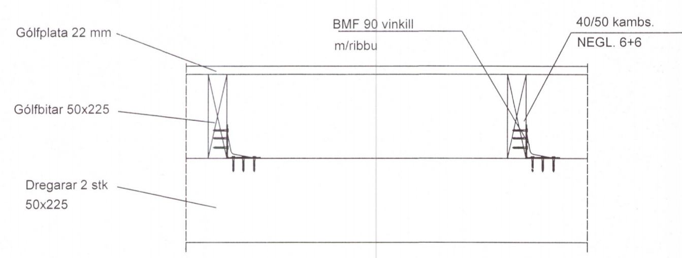
Festing dregarar/gólfbitar 1:10
