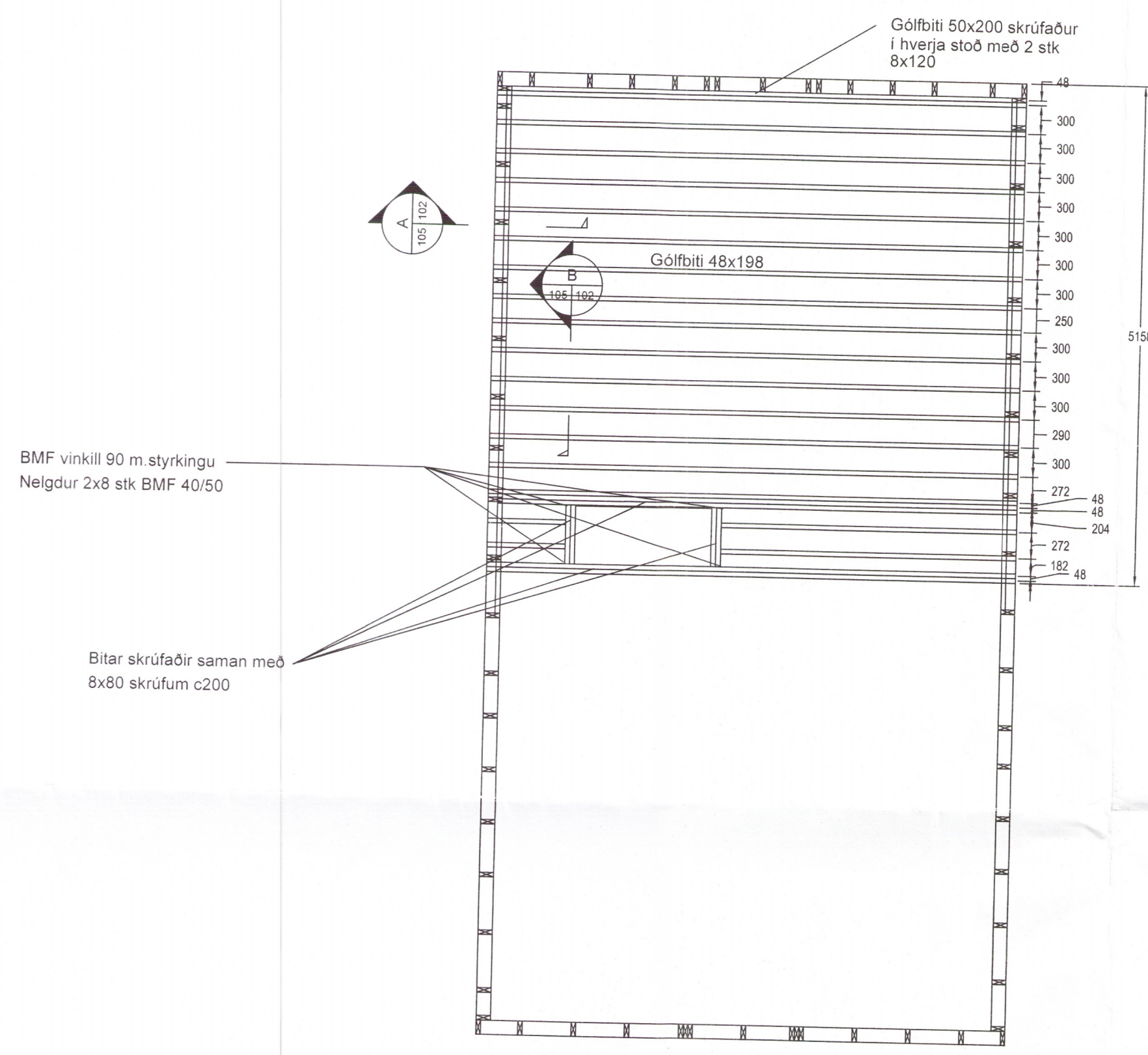
Gólfbitar í millilofti 1:50
