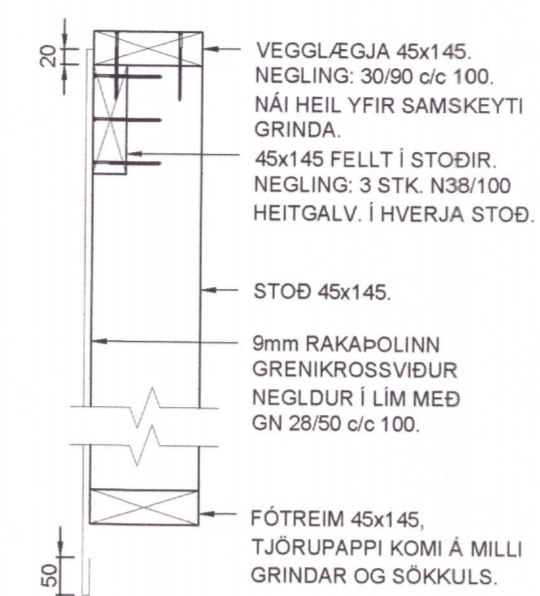
SNID Í GRINDUR Mkv 1:10
