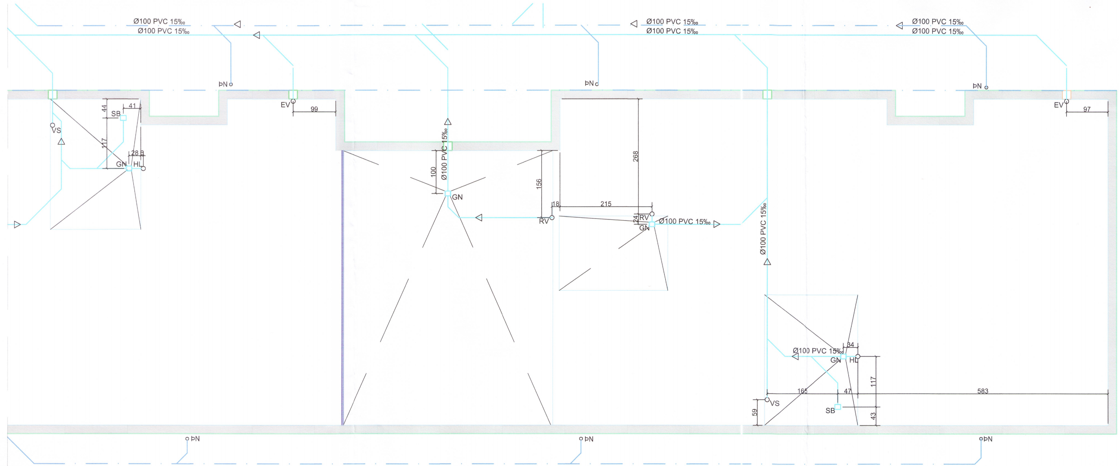
GRUNNMYND FRÁRENNSLI
