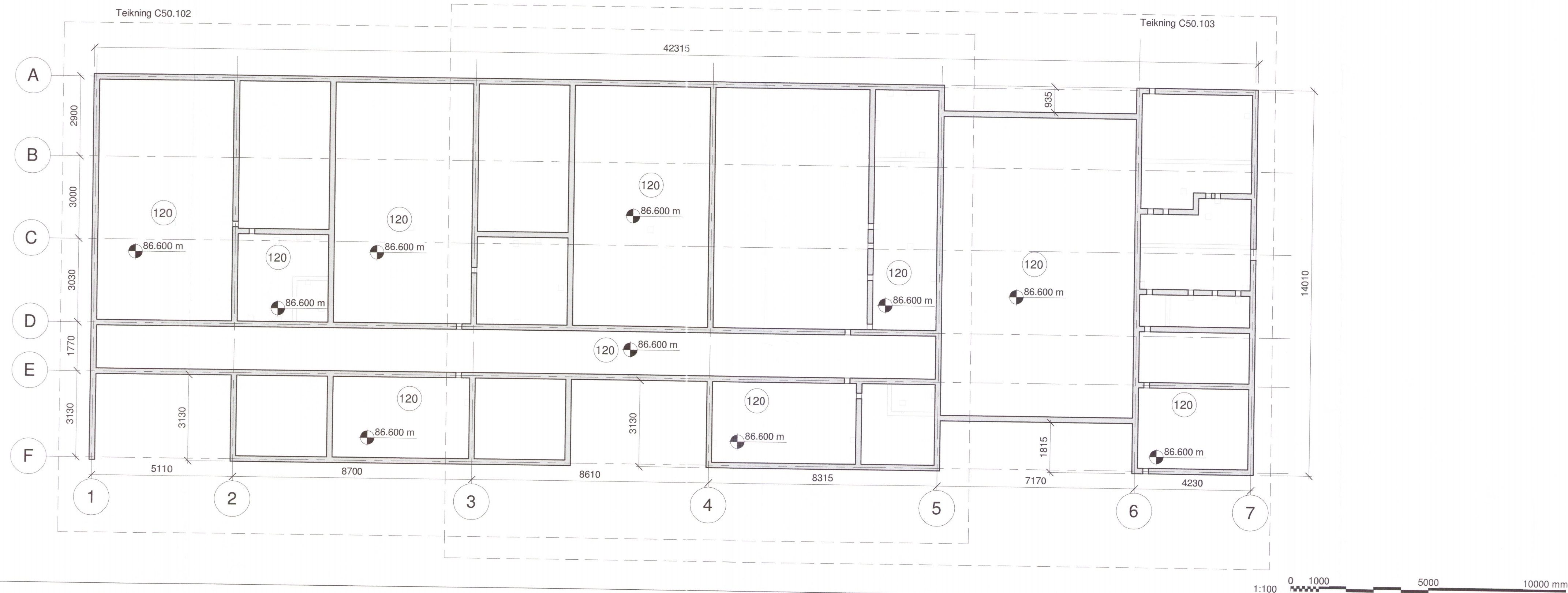
Grunnmynd - Undirstöður - Yfirlitsmynd 1 : 100
