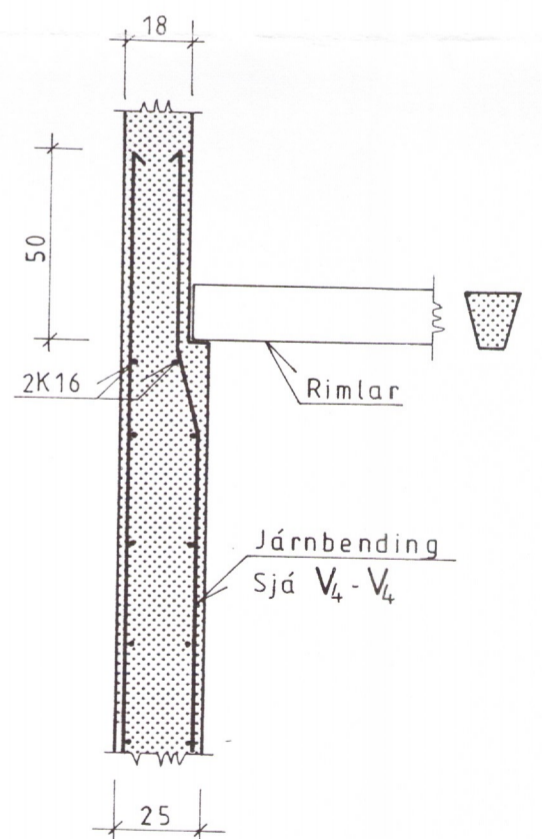
Snid V5-V5 M=1:20
