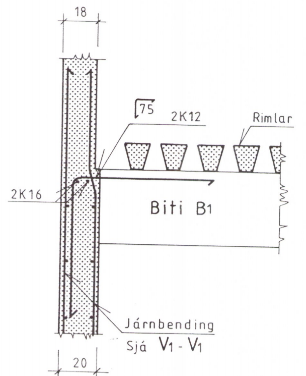
Snid V2-V2 M=1:20
