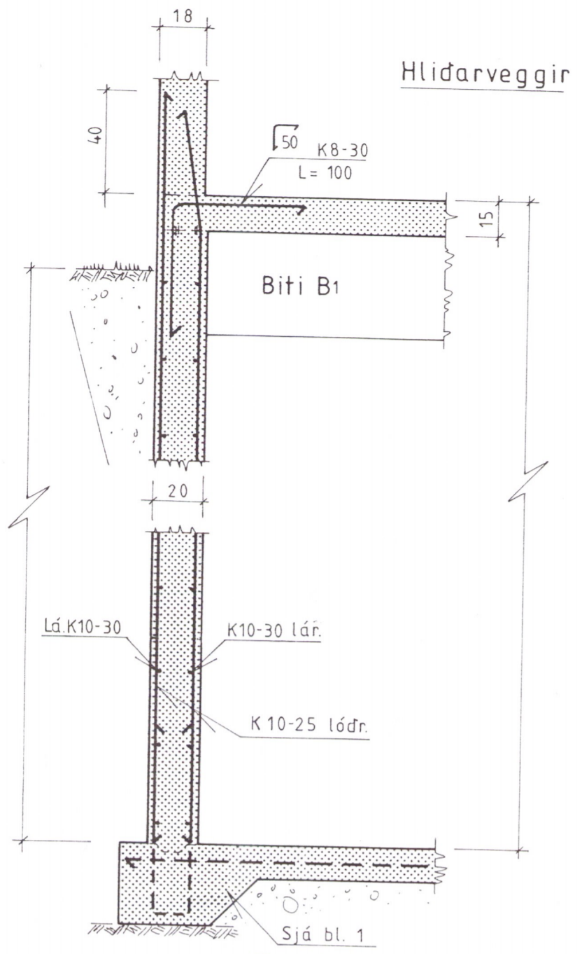
Snid V1-V1 M=1:20
