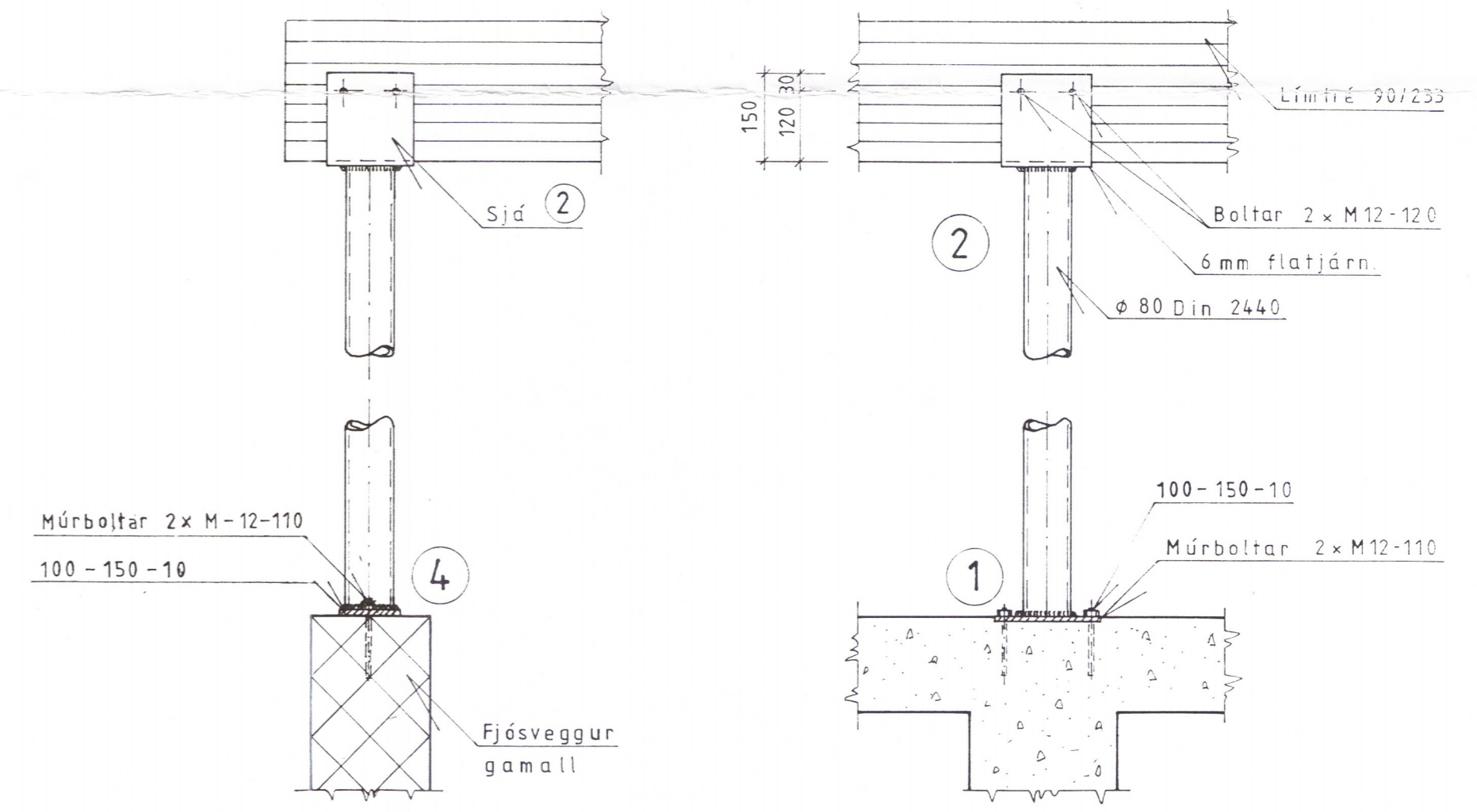
Öll deili M=1:10
