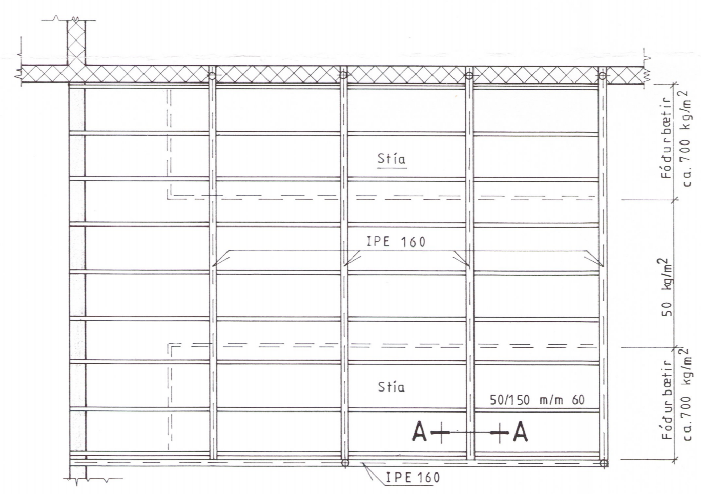
Möguleg fóðurgeymsla yfir mjaltabás M=1:50
