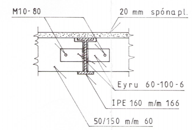
Snid A-A M=1:10
