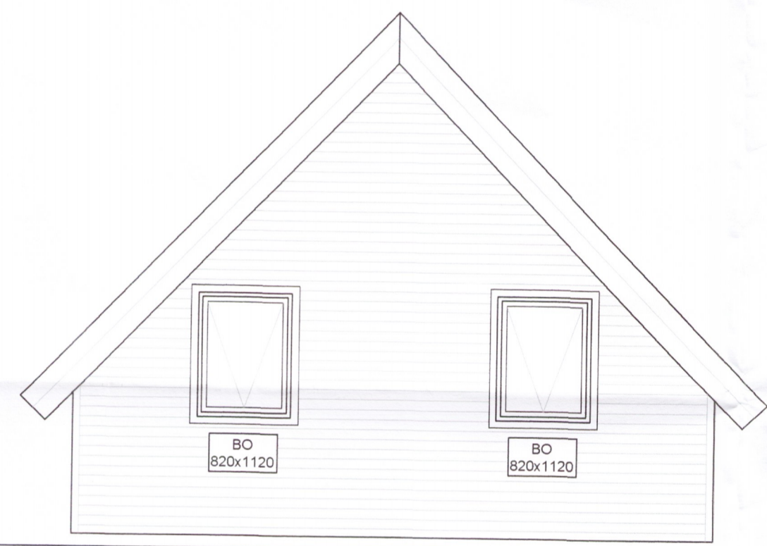
ÚTLIT NORÐAUSTURGAFL Mkv. 1:50
