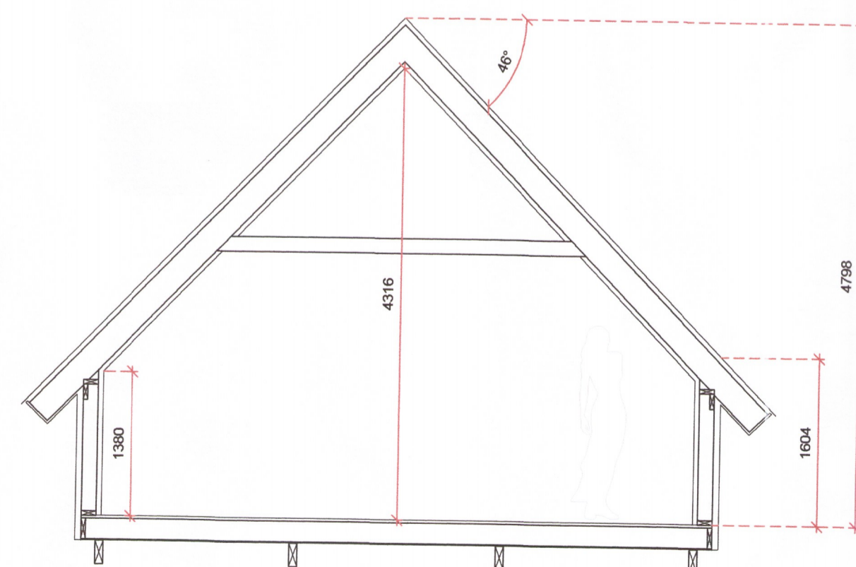
SNIÐ A2 Mkv. 1:50
