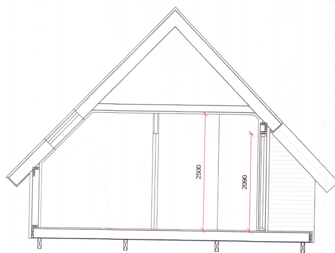
SNIÐ A1 Mkv. 1:50
