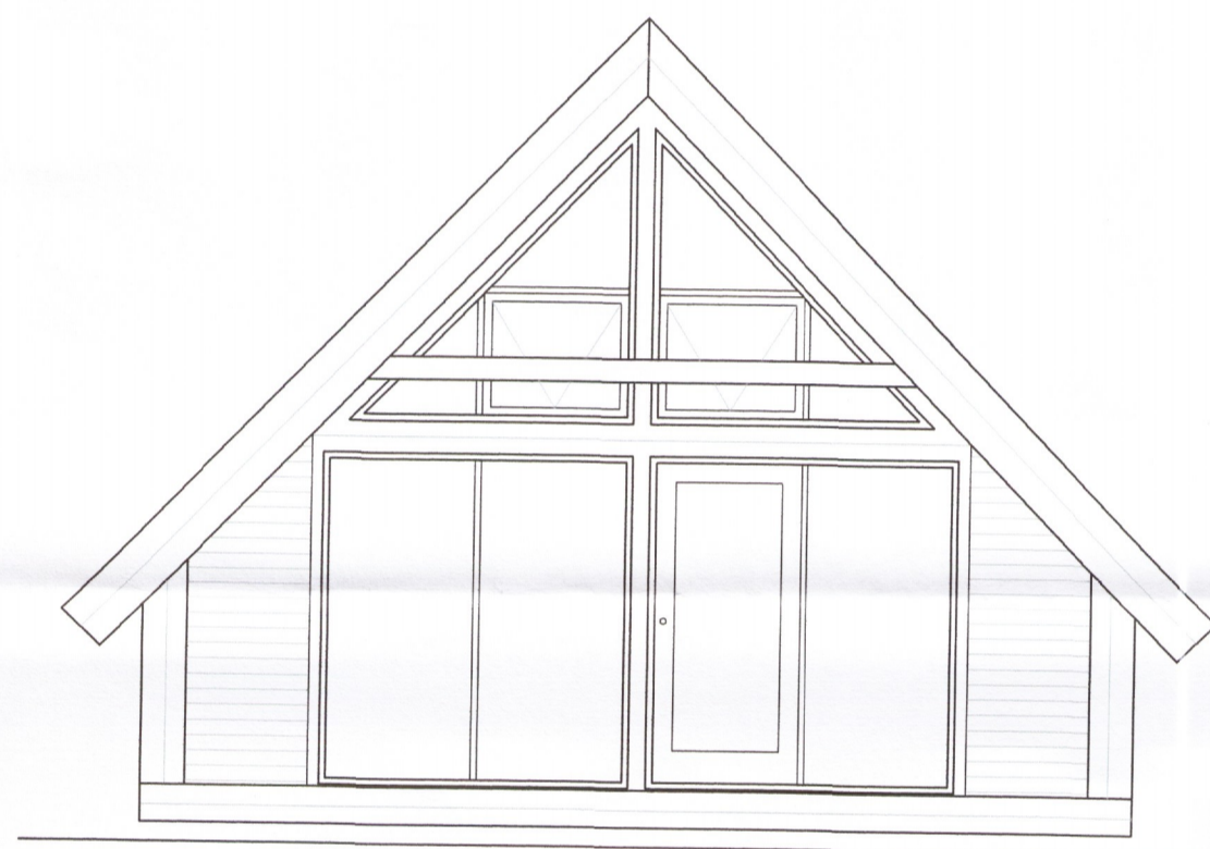
ÚTLIT SÚÐVESTURGAFL Mkv. 1:50
