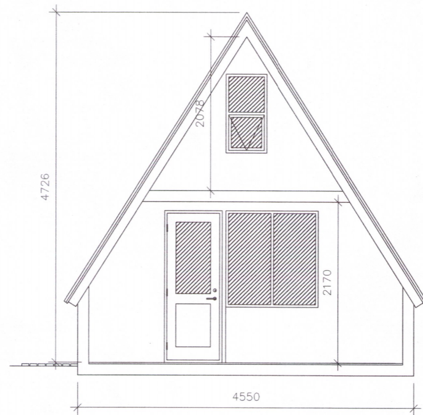
Sneiðing M1:50
