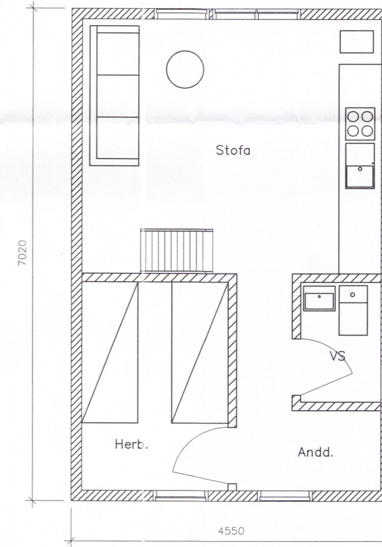
Grunnmynd M 1:50
