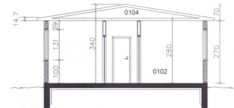
sneiðing B-B salerni
