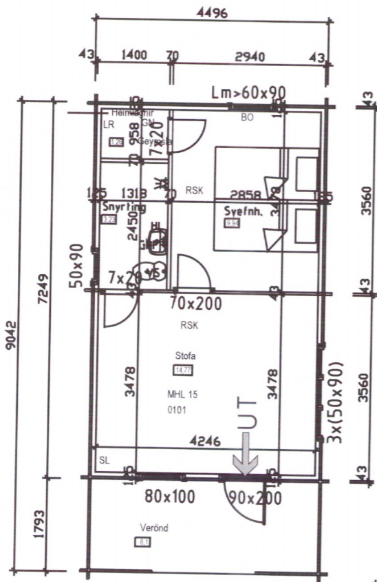
Grunnmynd
