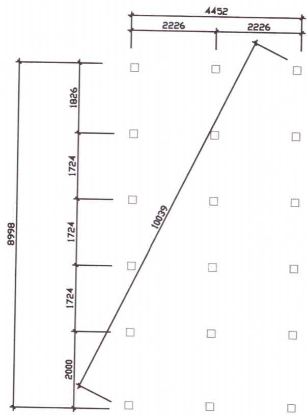
Undirstöður
